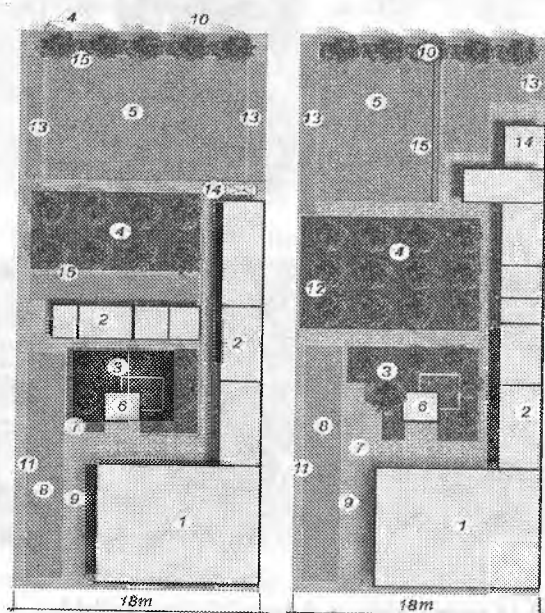
4.16-rasm. An'anaviy hovli maydonini obodonlashtirish bo'yicha takliflar: a) cho'l va dasht zonasi uchun mo'ljallangan hovli; b) qulay iqlimli vodiya va tog' vohalariga mo'ljallangan hovli; 1-turar joy uyi; 2-xo'jalik va maishiy imoratlar; 3-hovli; 4-mevali bog'; 5-sabzavot va poliz ekinlari; 6-chorpoya; 7-bolalar o'ynaydigan joy; 8-uzum ishkomi; 9-avtomashina joyi; 10-jiyda, bodom va boshqa daraxtlar; 11-berk devor; 12-pastqam to'siq; 13-yashil devor; 14-go'ng saqlash joyi; 15-ariq
