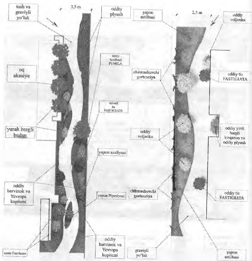
1.12-rasm. Dendroloyiha ishchi chizmalari.
