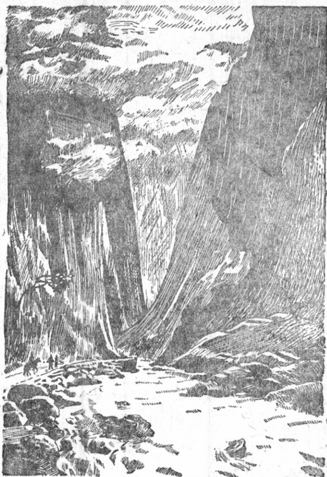
[Rəs. 15. Kavkaz taqlirida Darjəl çirəsi. Terek dərjəsi.
