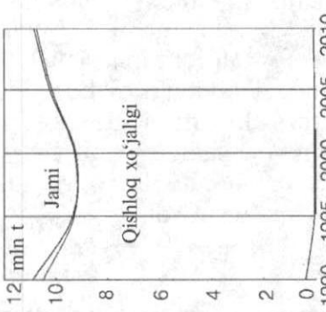
Ugl'erod qo'shoksidi emissiyasi bashorati
