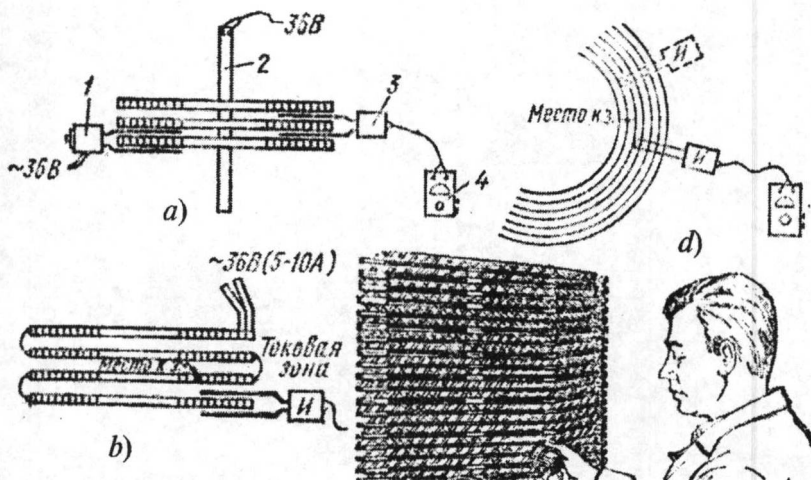
9.3-rasm. Kuch transformatorlari chulg'amlari o'ramlaridagi qisqa tutashuv joyini aniqlash:
