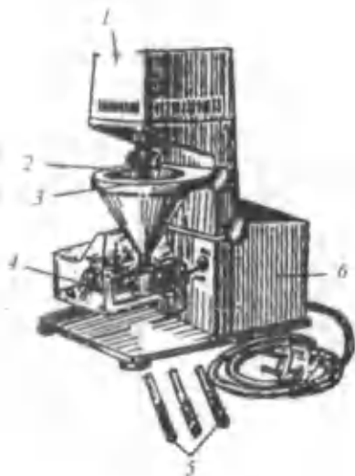
20-rasm. DVA-1,5 dozlash apparati.
