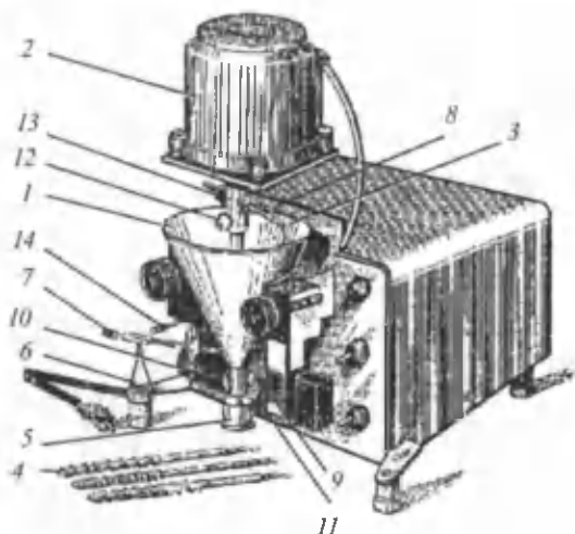
19-rasm. DP-2 dozlash apparati.
