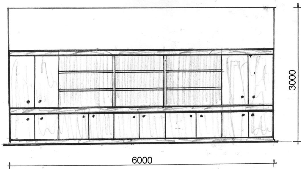
159-shakl. Sinf orqa devorining yoyilmasi (variant)
