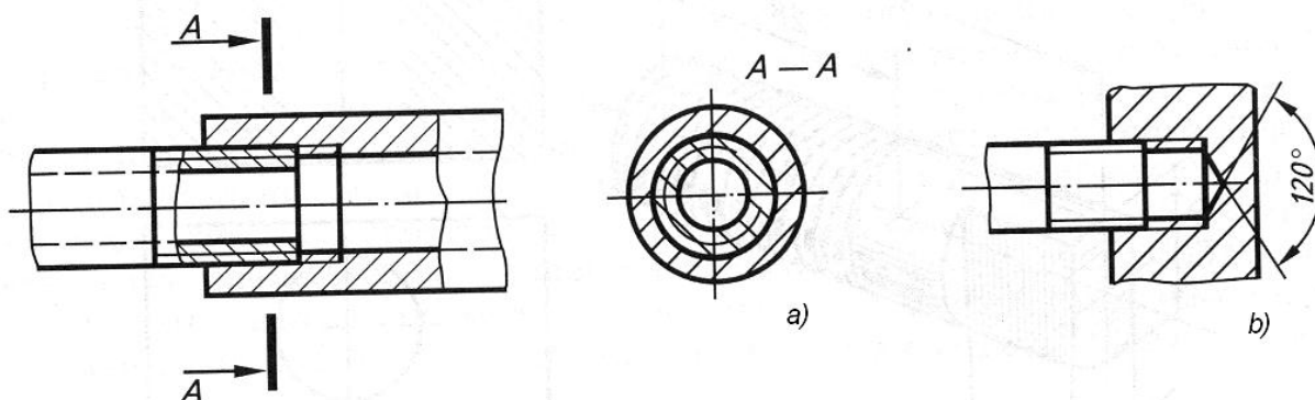
119-shakl. Rezbali birikmalarning tasvirlari
