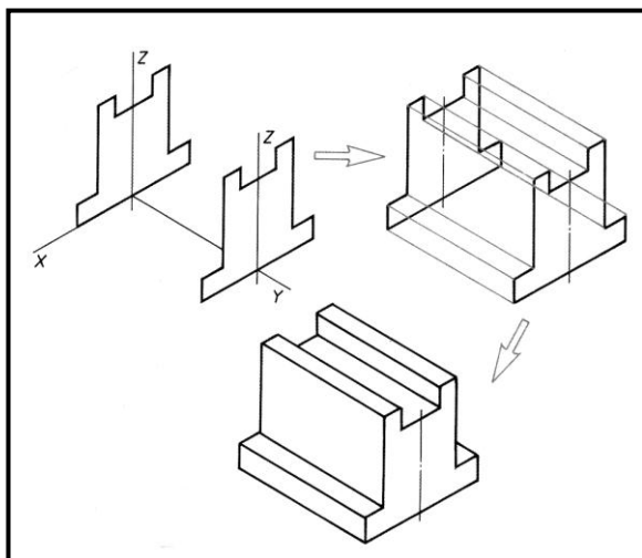
75-shakl. Shakl hosil qiluvchi yassi figuradan boshlab aksonometriya qurish
