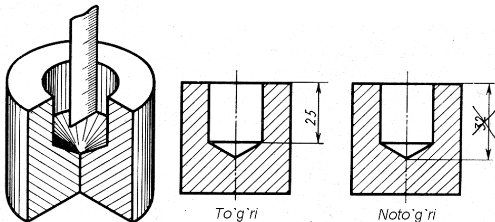
148-shakl. Parmada o`yilgan teshik chuqurligi o`lchamini qo`yish
