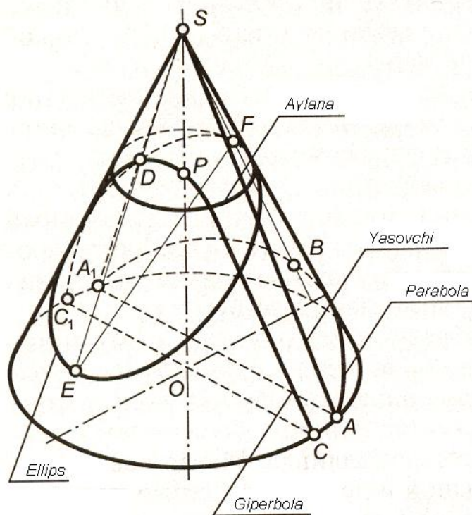
44—shakl. Lekalo egri chiziqlarinig hosil bo`lishi
