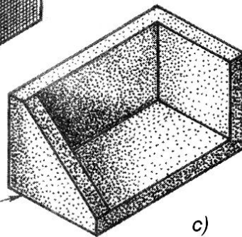
86-shakl. Texnik rasmda hajmni ko`rsatish: a) shatirovka, b) shraffirovka, s) nuqtali soylash usullariga misollar
