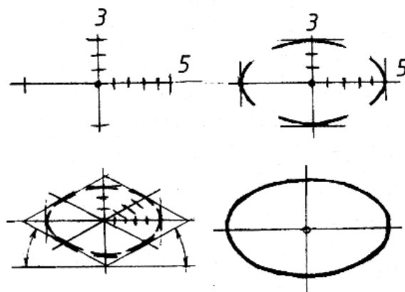
82-shakl. Aylanani izometriyada yasash bosqichlari
