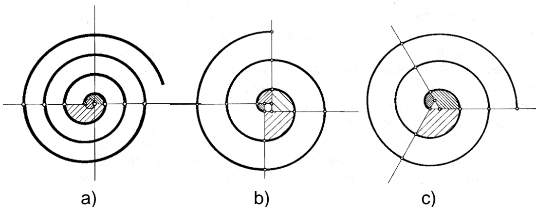
41-shakl. Lekalo yordamida bajarilgan ikki (a), to'rt (b) va uch (s) markazli o'ramlar
