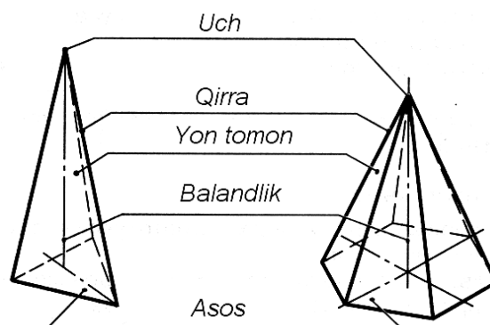
108-shakl. Piramida va uning elementlari
