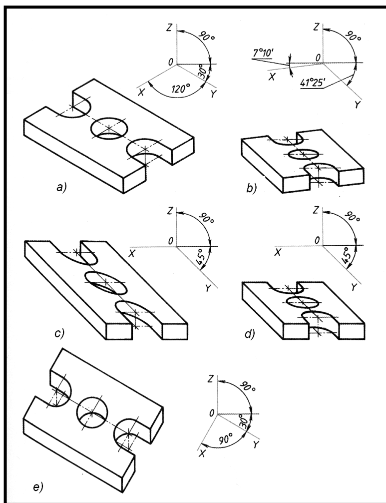
68-shakl. DST 2.317-69 tomonidan belgilangan aksonometrik proeksiyalar a) to`g`ri burchakli izometrik proeksiya; b) to`g`ri burchakli dimetrik proeksiya; c) qiyshiq burchakli frontal izometrik proeksiya; d) qiyshiq burchakli frontal dimetrik proeksiya; e) qiyshiq burchakli gorizontal izometrik proeksiya
