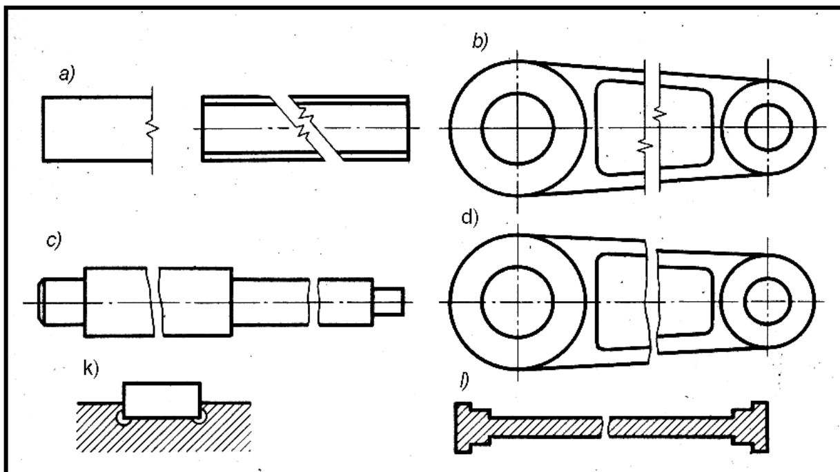
62-shakl. Uzun detallarni uzib tasvirlanishi
