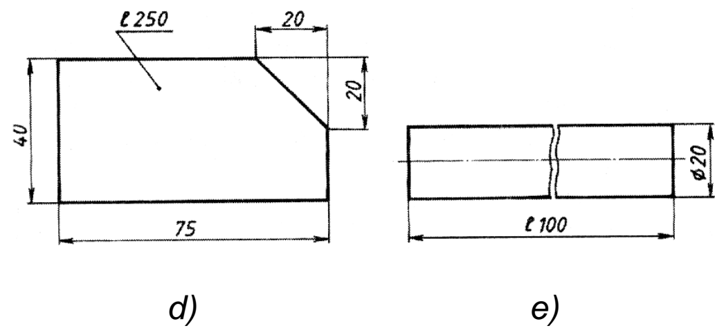
57-shakl. O'lchamlarning klassifikatsiyasiga misollar: bir tekis joylashgan elementlarning (a - chiziqli, b - burchakli), s - gabarit va d -, e - detal uzunligi o'lchamlarini qo'yish
