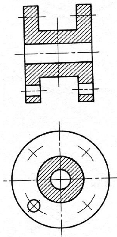
67-shakl. Detaldagi bir xil teshiklar simmetrik joylashgan hollarda chizmada tasvirlanishi
