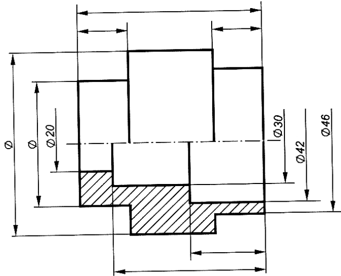
60-shakl. O'lcham qo'yish variantlariga misollar
