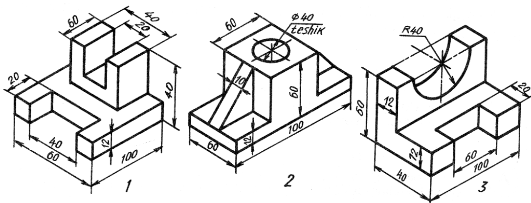
49-shakl. Bosh ko`rinishni aniqlash misoliga na'munalar
