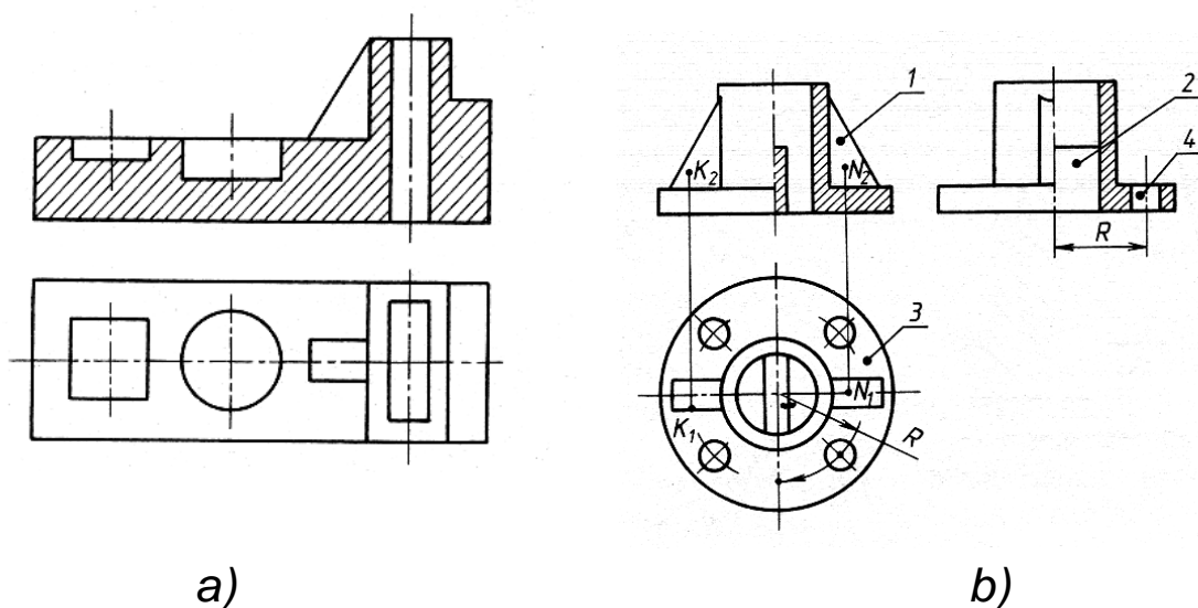
65-shakl. Kesuvchi tekislikda joylashgan yupqa devorlarni chizmada tasvirlash
