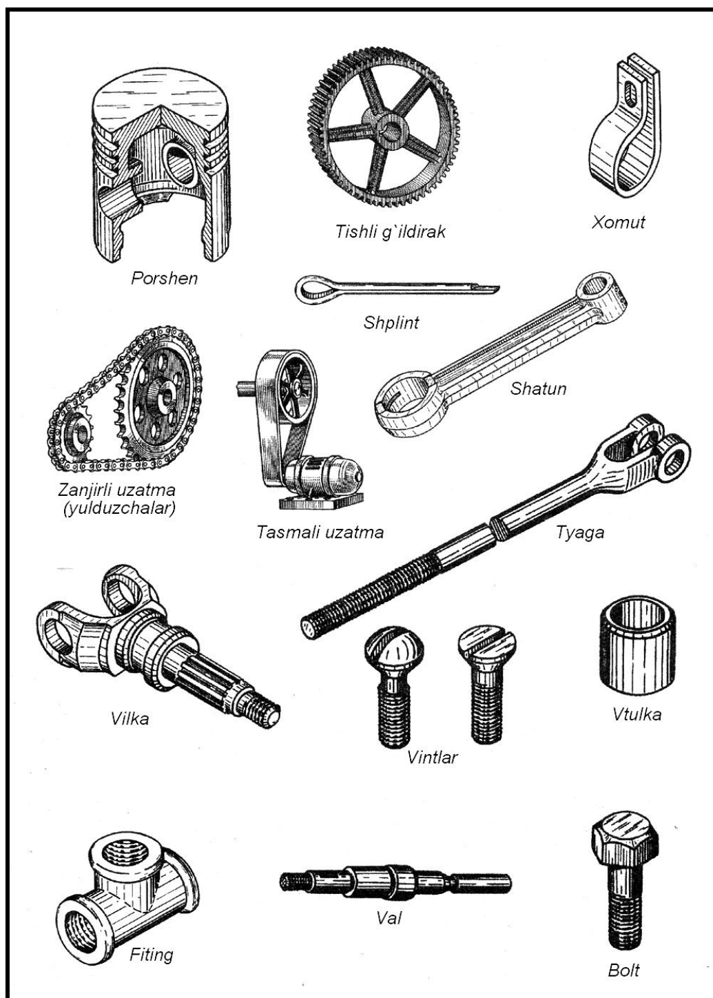
113-shakl. Tipaviy detallar va uzatmalariga misollar plakati
