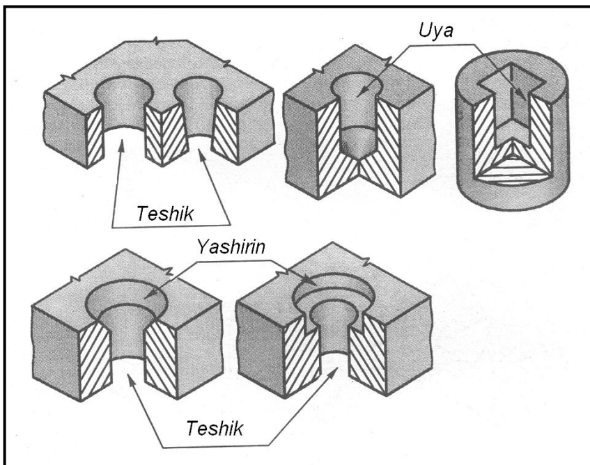
179-shakl. Teshik – detaldagi silindrik, konik yoki qirrali o`tish (teshik). Teshiklar ochiq yoki berk, silliq yoki rezbali, uzunligi bo`yicha o`zgarmas yoki pog`onali bo`ladi.
