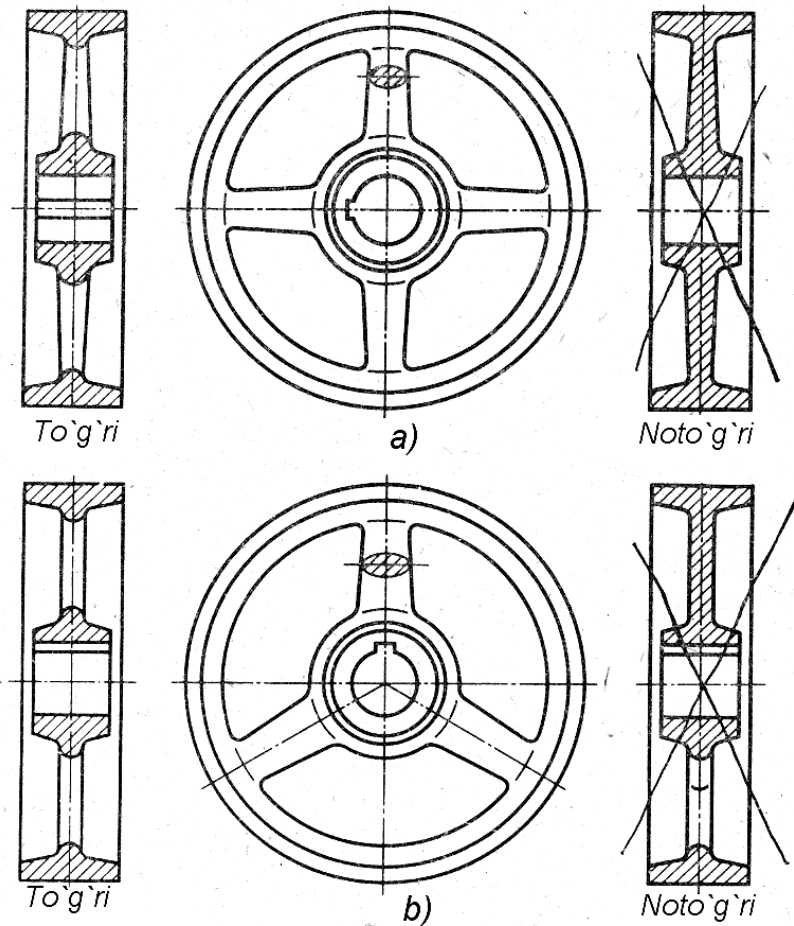
146-shakl. Kegayli shkiv qirqimi
