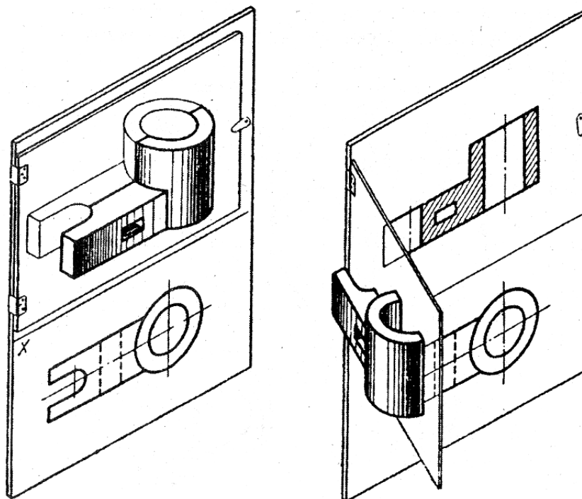
13-shakl. Qirgim hosil bo`lishini namoyish qilish uchun dinamik plakat
