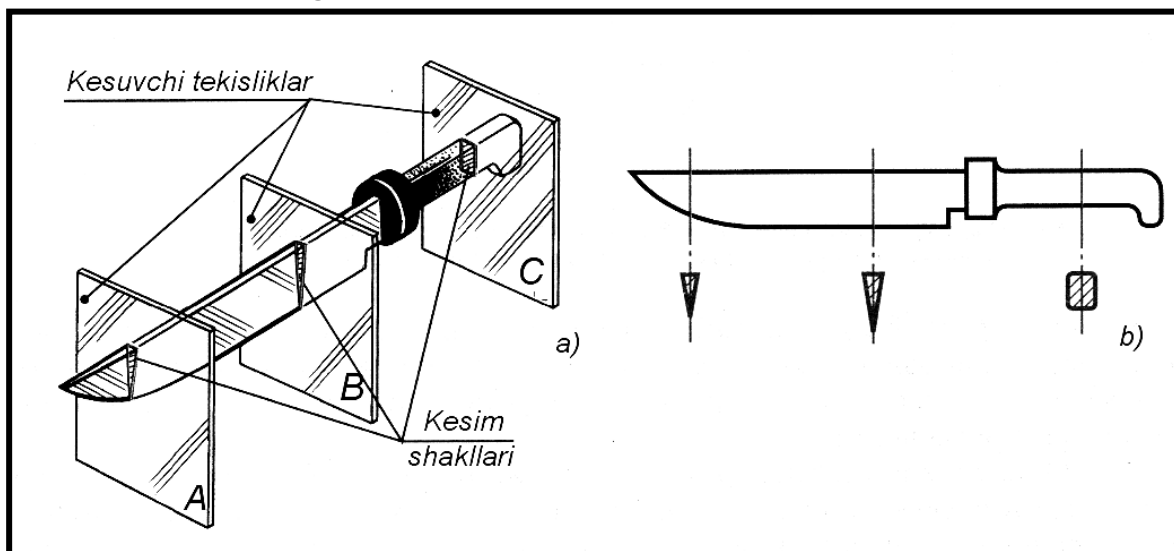
91-shakl. Kesimning hosil bo'lishi
