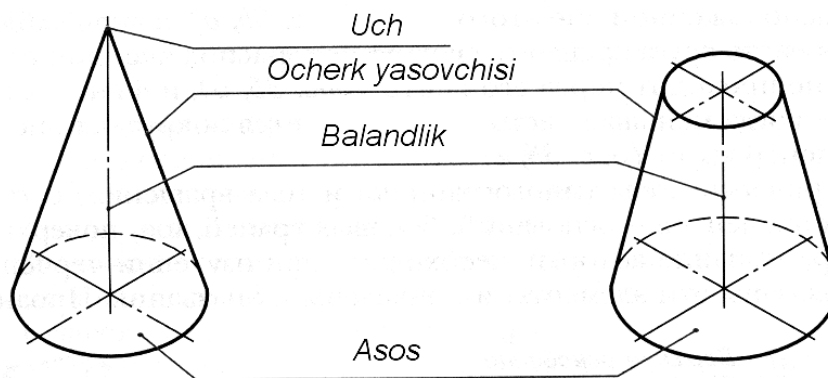
110-shakl. Konus va uning elementlari
