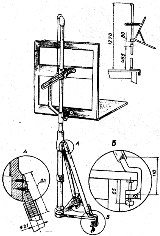
18-shakl. Uch tomonli burchak modeli (B.V.Budasov konstruksiyasi)
