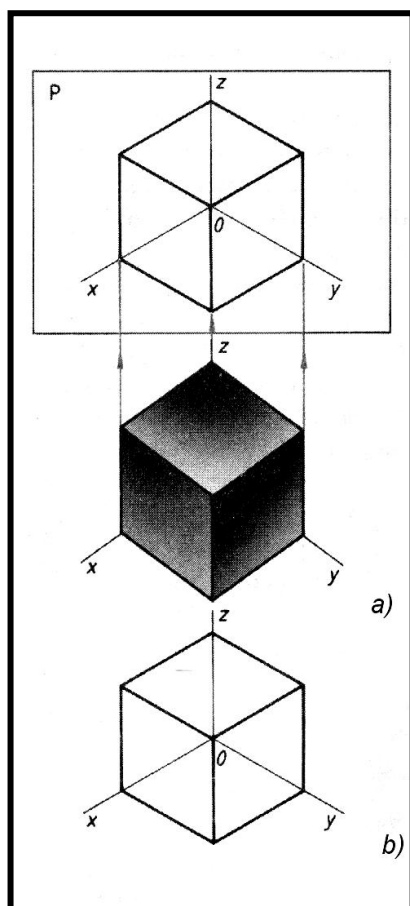
72-shakl. To`g`ri burchakli izometrik proeksiyaning hosil bo`lishi
