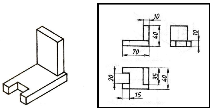
47-shakl. Proeksiyalashni tushuntirishga misol
