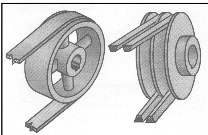
197-shakl. Shkiv – enli gardishli g`ildirak ko`rinishidagi tasmali uzatma tarkibiga kiruvchi detal.
