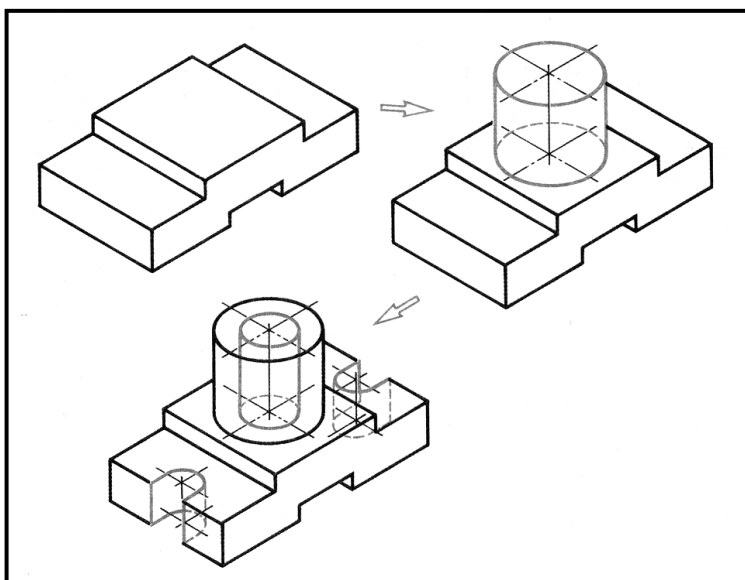
78-shakl. Kombinatsiyalashgan usul yordamida detal izometrik proeksiyasini qurish
