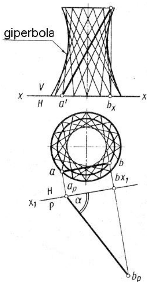
37-shakl. Kojux sirtini loyihalashda tashilayotgan material traektoriyasini hisobga olishga misol
