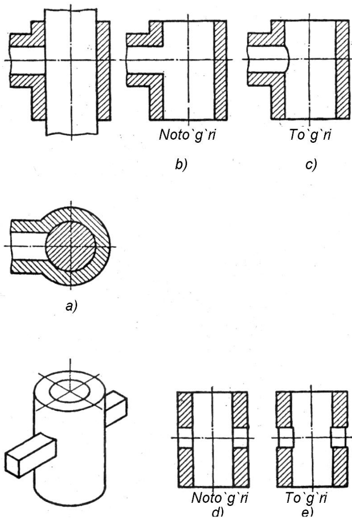
150-shakl. Yig`ish chizmalarini detallarga ajratishda o`quvchilar yo`l qo`yadigan tipik xatolarga misollar
