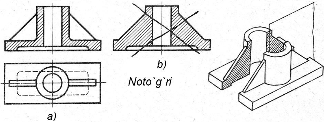
145-shakl. Yupqa qovurg`a bo`ylab qirqim yasash
