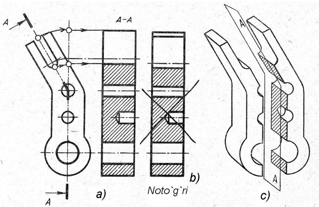
147-shakl. Murakkab qirqimning chizmada tasvirlanishi
