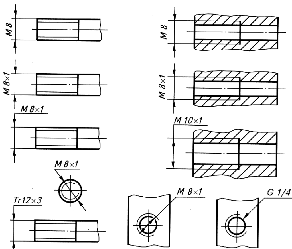
118-shakl. Chizmada rezbalarning tasvirlanishiga misollar
