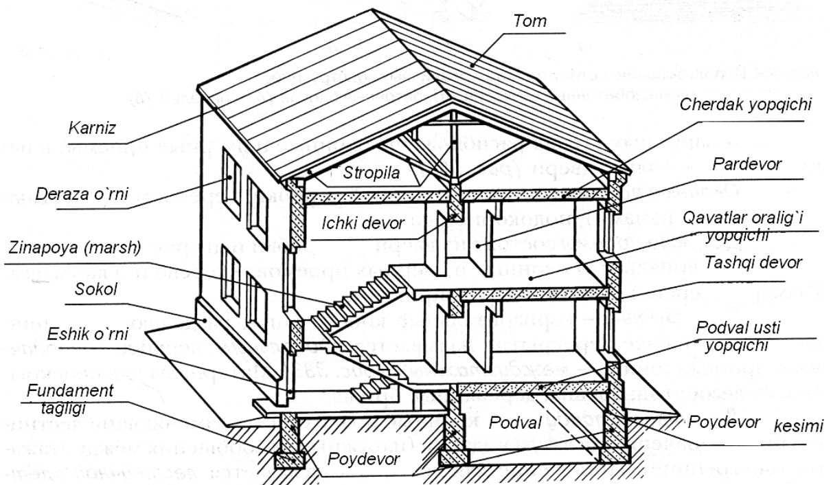
124-shakl. Binoning konstruktiv elementlari
