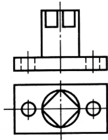
102-shakl. "Tayanch" detali chizmasi
