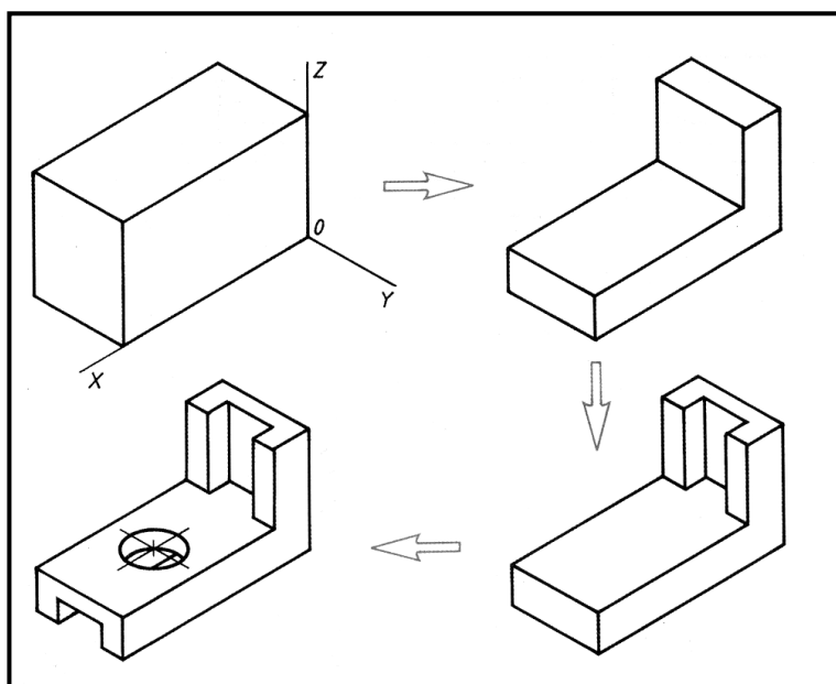
76-shakl. Ketma-ket qirqish usuli bilan aksonometriya yasash
