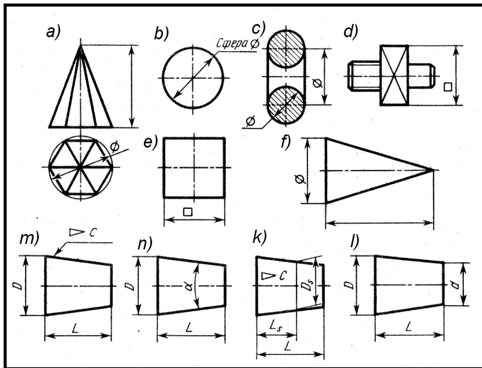
61-shakl. Chizmalardagi shartlilik va soddalashtirishlar
