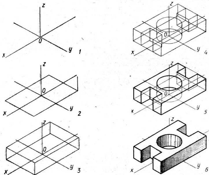
87-shakl. Texnik rasmni bajarish bosqichlari
