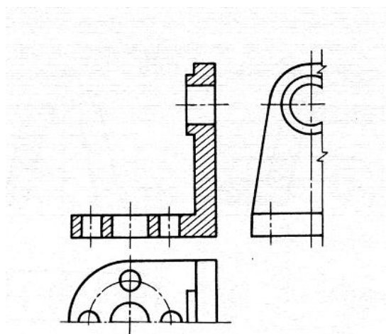
63-shakl. Agar tasvir simmetrik bo`lsa, standart tasvirning yarmini yoki sal ko`proq`ini tasvirlashga ruxsat beradi
