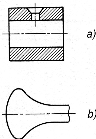
65-shakl. Kesuvchi tekislikda joylashgan yupqa devorlarni chizmada tasvirlash
