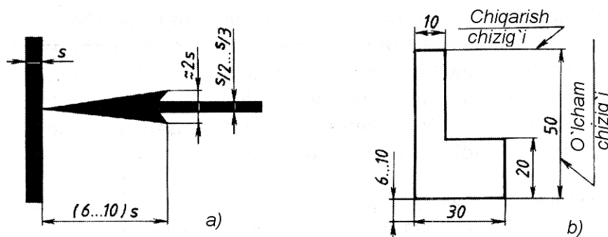
56-shakl. Chiziqli o'lcham qo'yish tartibi
