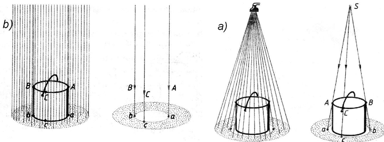
46-shakl. Proeksiyalar hosil bo`lishini tushuntirishga misollar: a) markaziy proeksiyalash; b) parallel proeksiyalash
