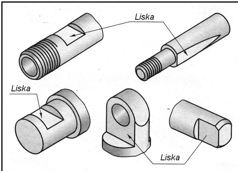
178-shakl. Liska – detalning silindrik, konik va sferik uchaskalaridagi yassi kesik. Odatda liska sirti detal geometrik o`qiga parallel bo`ladi.
