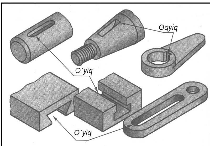
180-shakl. O`yiq – odatda detal geometrik o`qi bo`ylab bajarilgan chuqurcha. Shakli va ishlatilish soha-siga ko`ra turli konstruktiv shaklda bo`ladi.
