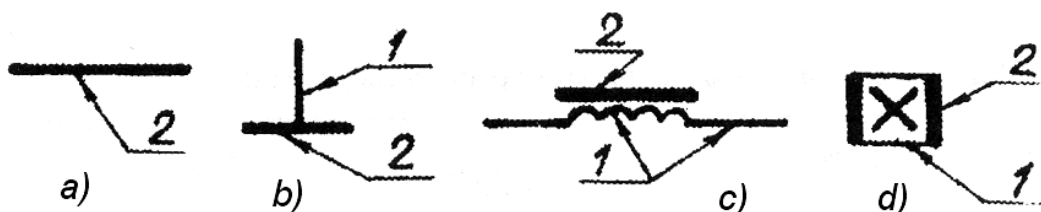
122-shakl. Elektr sxemalaridagi shartli belgilashlar:
