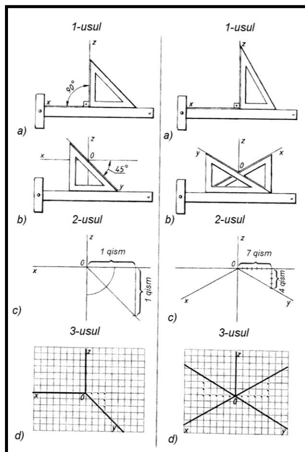
73-shakl. Aksonometriya o`qlarini qurish usullari
