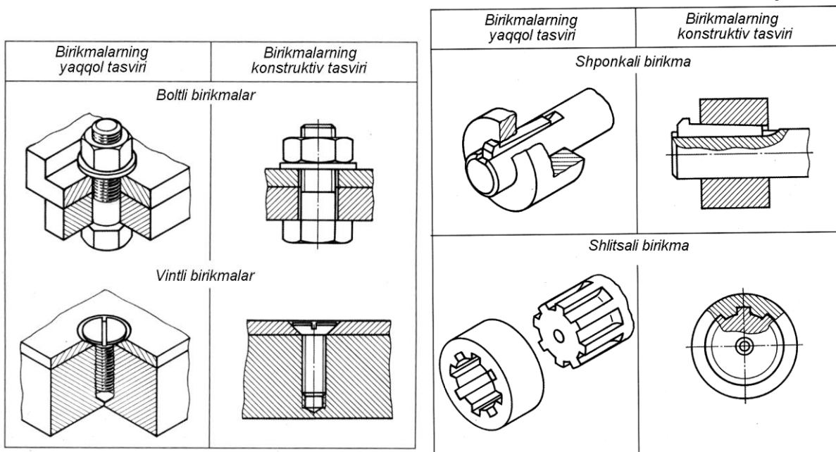
114-shakl. Ajraladigan birikmalarning yaqqol tasviri va chizmada tasvirlanishini tushintirishga oid plakat namunasi
