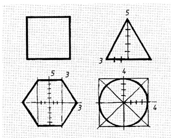
81-shakl. Yassi figuralar texnik rasmini bajarish usullari
