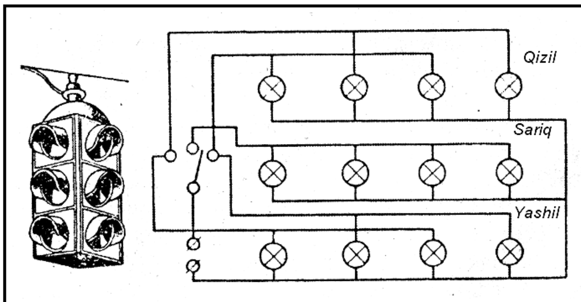
121-shakl. Svetoforning prinsipial elektr sxemasi plakati
