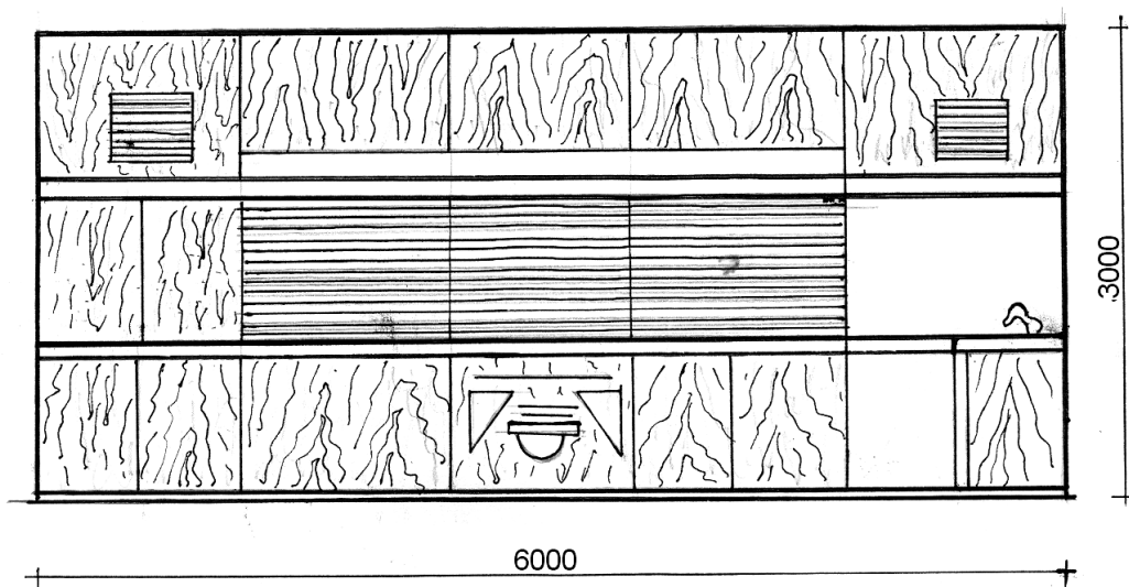
157-shakl. Sinf oldingi devorining yoyilmasi (variant)
