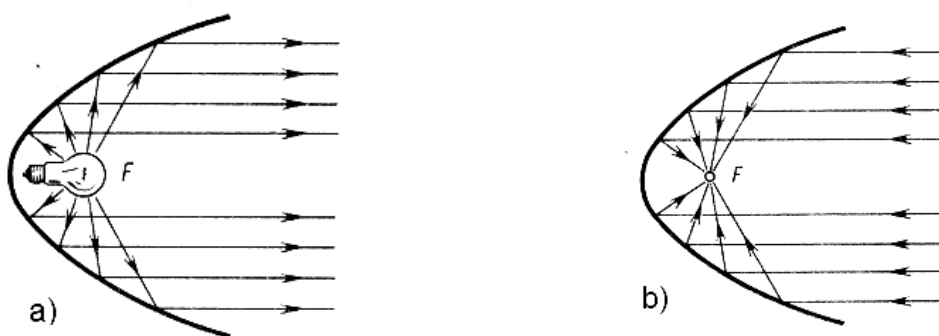
45-shakl. Parabolik qaytargichlarning amaliyotda qo`llanilishiga misollar: a) yoritish asboblarda; b) teleskop, radiolokator va antennalarda
