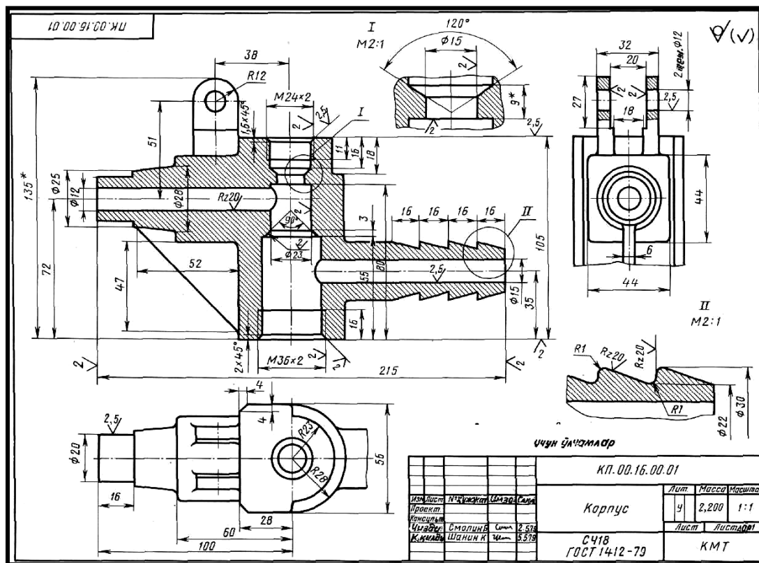
22-shakl. Zamonaviy mashinasozlik chizmasi
