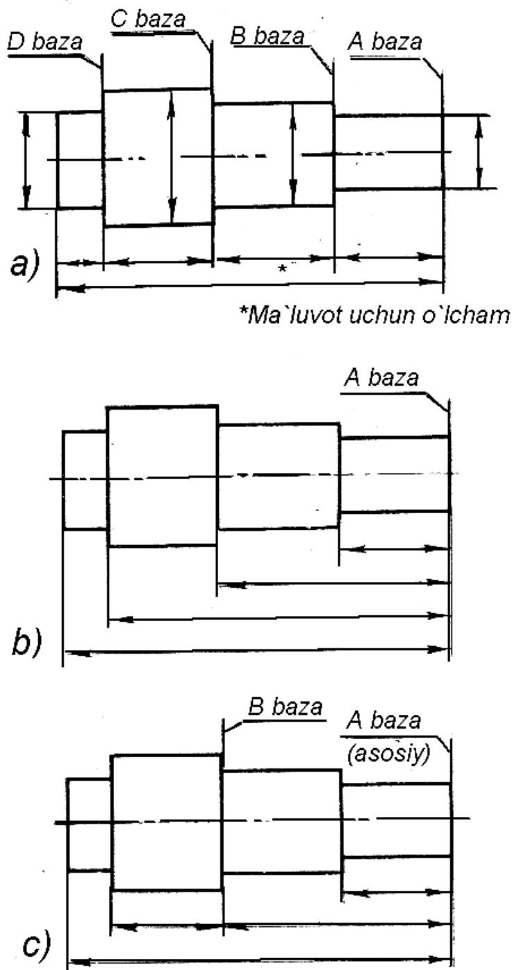
58-shakl. O'lcham qo'ish usullari: a) zanjirsimon; b) koordinalali; s) kombinatsiyalashgan (aralash)
