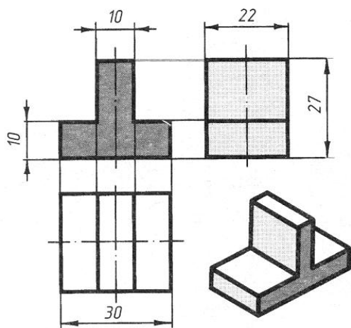
50-shakl. Yaqqol tasvir bo`yicha ko`rinishlarni bajarish
