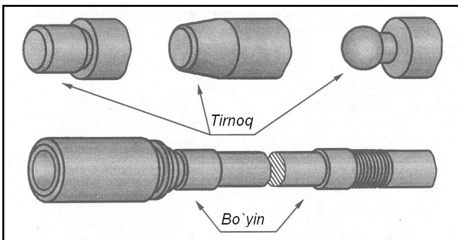
196-shakl. Tirnoq (ship) – detallarni o`zaro biriktirish uchun mo`ljallangan chiqiq.
