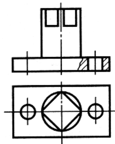
104 -shakl. Tayanchning mahalliy qirqim bilan bajarilgan chizmasi
