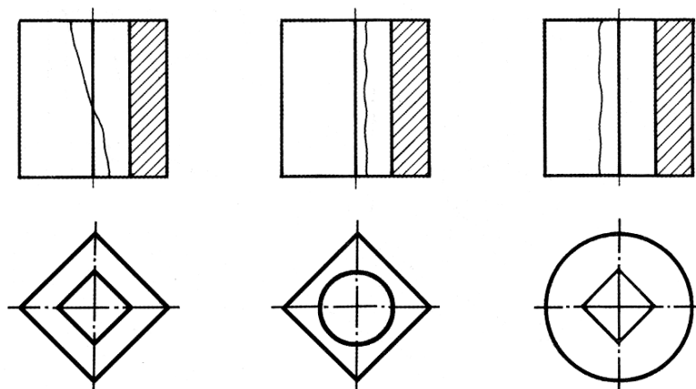
105-shakl. Ko`rinishning bir qismi va qirqimning bir qismini birlashtirib tasvirlashning xususiy hollariga misollar
