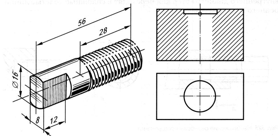
119-shakl. Rezbali birikmalarning tasvirlari
