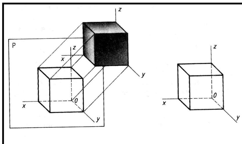
71-shakl. Qiyshiq burchakli frontal dimetrik proeksiyaning hosil bo`lishi
