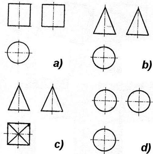
53-shakl. Proeksiyalari bo`yicha geometrik jismlarni aniqlash
