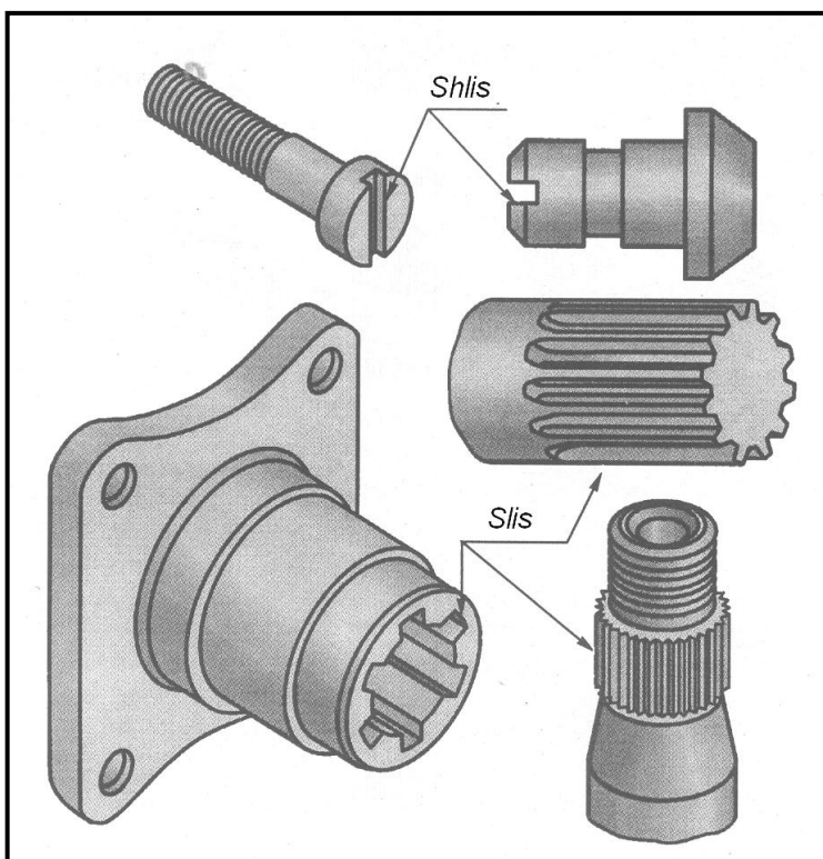
198-shakl. Shlis – ikkita ma`noda qo`llaniladi: 1 – vint kallagidagi otvertka uchun qilingan ariqcha yoki chuqurcha; 2 – shlisalar – tishli (shlisali) birikmaning konstruktiv xususiyati.
