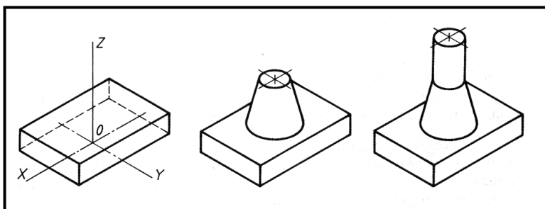
77-shakl. Qismlarni o'rtirib borish usuli bilan aksonometriya yasash
