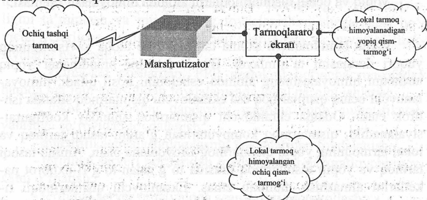
8.14 -rasm. Uchta tarmoq interfeysli bir brandmauer asosida yopiq va ochiq qismtarmoqlarni alohida himoyalash sxemasi.
