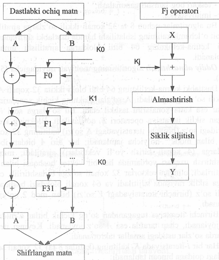
5.14-rasm. Oddiy almashtirish algoritmidagi shifrlash jarayonining blok-sxemasini.
