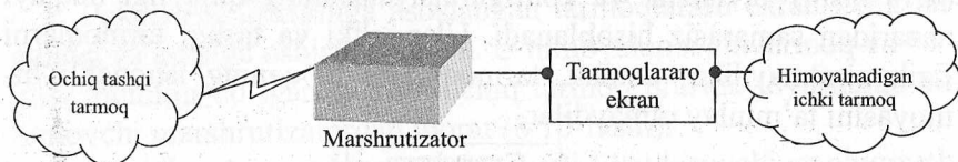
8.12-rasm. Lokal tarmoqni umumiy himoyalash sxemasi.
