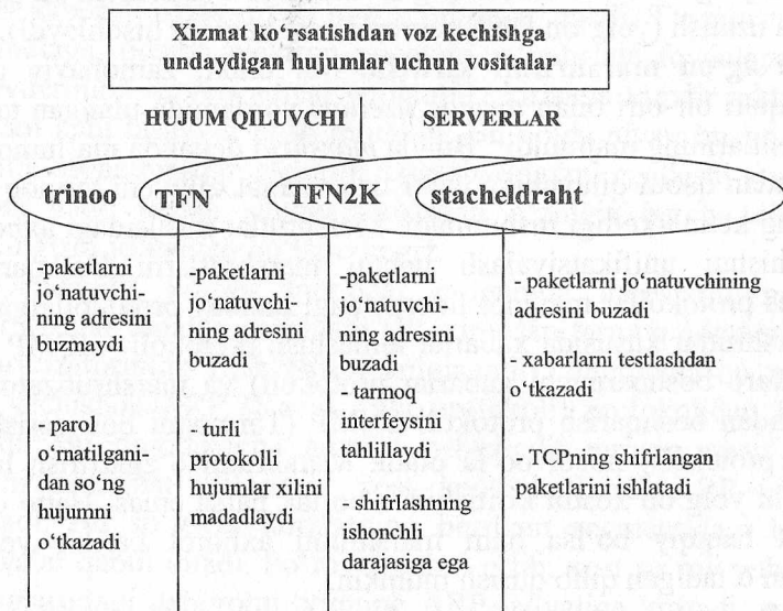
2.1-rasm. Xizmat qilishdan voz kechishga undaydigan hujum vositalarining xarakteristikallari.
