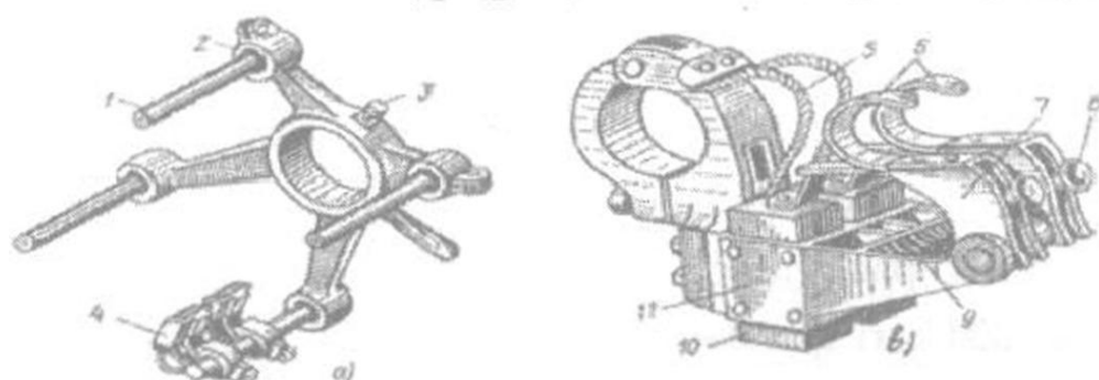
5.4-rasm. O'zgarmas tok mashinasining chutka mexanezmi: a – traversa; b – cho'tka tutqich va cho'tkalar: 1 – cho'tka tutqichni mahkamlash uchun izolatsiyalangan barmoq; 2 – barmoqni siquvchi kronshteyn; 3 – cho'tkalarning kollektortordagi holatini belgilash uchun bolt; 4 – cho'tka tutqich; 5 – sim; 6 va 7 – cho'tkani kollektorga siquvchi qismlar; 8 – cho'tka va kollektor orasidagi bosimni rostlash uchun gayka; 9 – prujina; 10 – cho'tka; 11 – cho'tkani o'rnatish uchun moslama.
