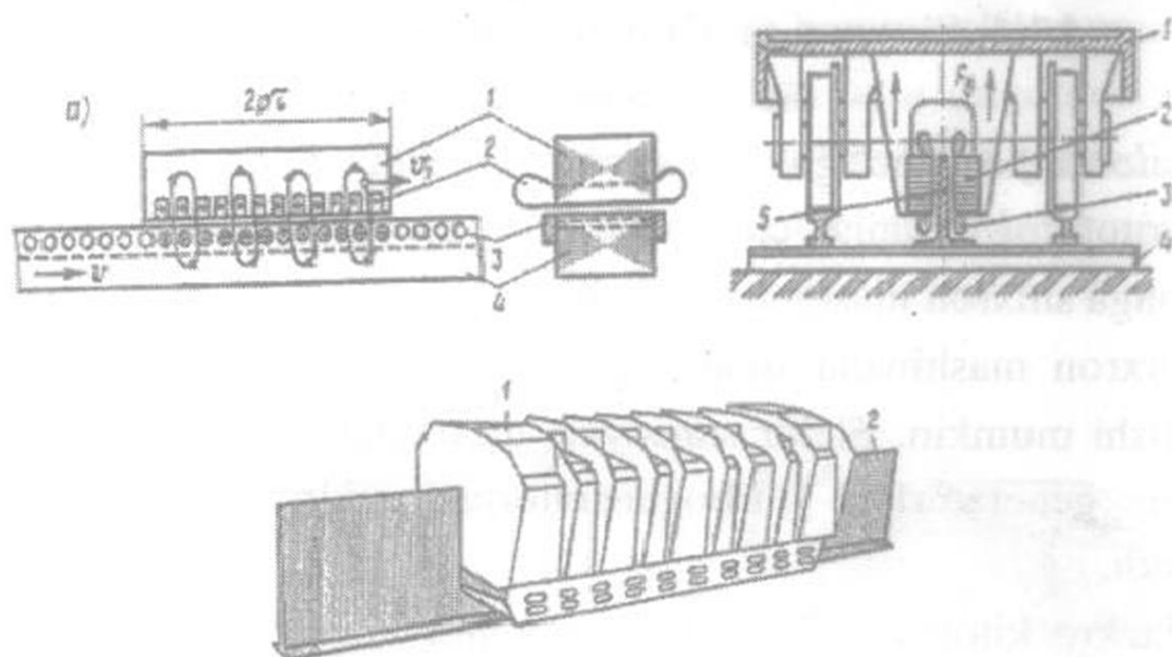
3.26-rasm. Chiziqli asinxron motorning: a - elektromagnit sxemasi (bunda: 1 - stator, 2 - uch fazali chulg'am; 3- qisqa tutashgan chulg'am, 4 - uzun po'lat o'zak) b-temir yo'l transportining harakatlanuvchi qismi(1) da o'rnatish sxemasi (bunda: 2 - stator, 3 - chulg'am; 4- uzun po'lat o'zak, 5-relslar orasida mahkamlash uchun moslama); c – umumiy ko'rinishi (bunda: 1 - stator, 2 - uzun po'lat o'zak).
