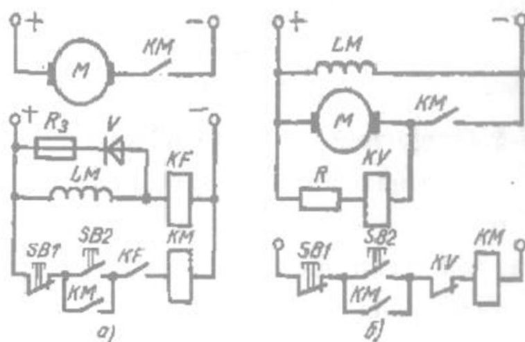
Rasm.7.15 O'zgarmas tok motorini maydonning yo'qolishidan (a), kuchlanishning oshib ketishidan (b) himoyalash sxemalari.
