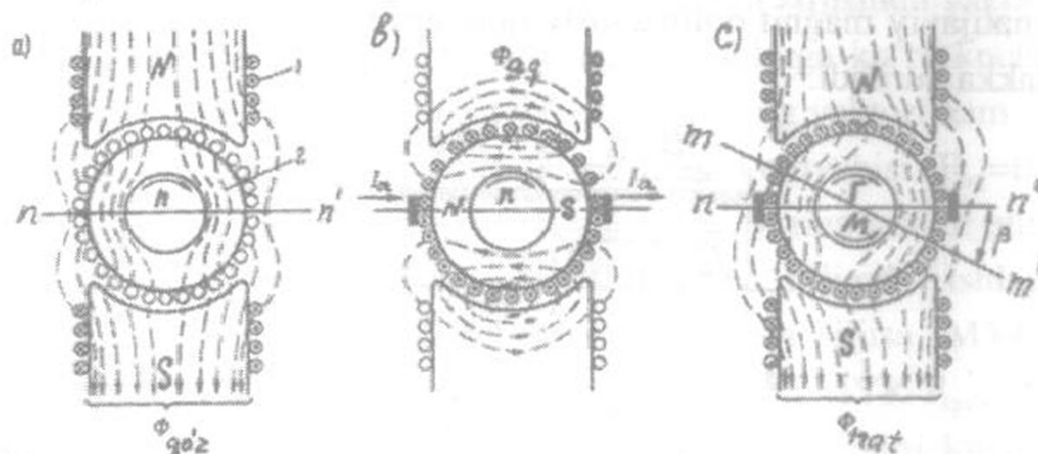
5.12-rasm. O‘zgarmas tok mashinasining magnit maydoni: a ) qo‘zg‘atish chulg‘amining maydoni F_{qo'z} , 1 – qo‘zg‘atish chulg‘ami, 2 – yakor; b ) yakor chulg‘amining maydoni F_a ; c ) mashinaning natijaviy magnit maydoni F_{nat}
