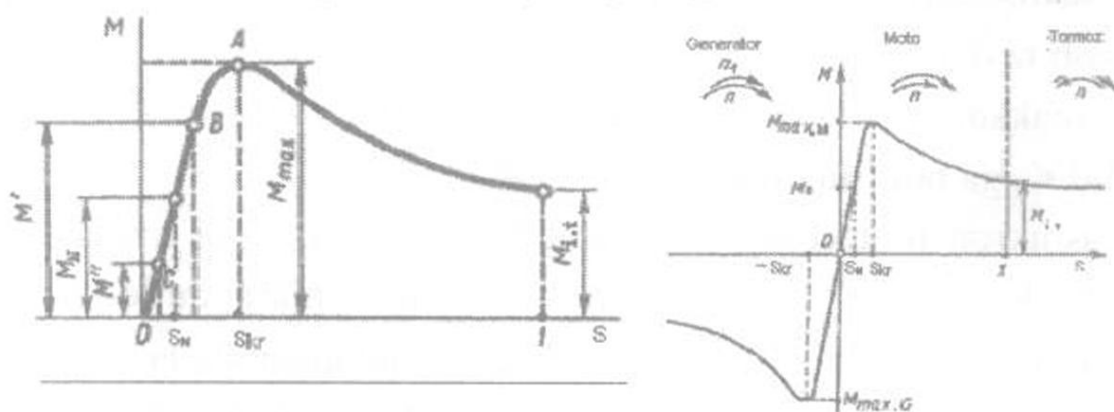
3.7-rasm. Asinxron mashinaning motor, generator va elektromagnit tormoz rejimlari uchun mexanik xarakteristiklari (a, b) - M_q f(s)
