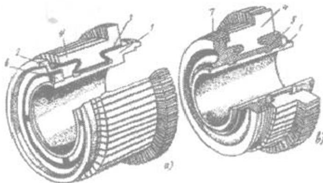
5.3-rasm. O'zgaras tok mashinasining metall (a) va plastmassa (b) korpusli kollektori: 1 – korpus; 2 – siquvchi flanets; 3 – izolatsion qistirma; 4 – kollektor plastinalari; 5 – plastmassa; 6 – siquvchi halqa; 7 – bandaj
