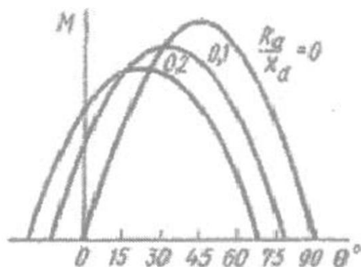
4.28-rasm. Kam quvvatli reaktiv sinxron motorning aktiv va induktiv qarshiliklari nisbati x_d/x_q ning har xil qiymatdagi burchak xarakteristikalari.
