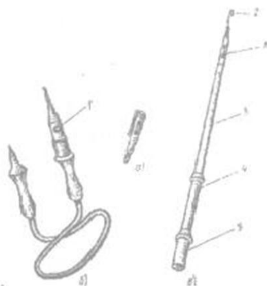
8.4- Rasm. Kuchlanish ko'rsatkichlari: a, b - 1000 V gacha kuchlanishli qurilmalarda, v - 1000 V dan katta kuchlanishli qurilmalarda; 1 - neon lampa, 2 - shchup, 3, 4 - ko'rsatkichning ishlaydigan va izolyatsiyalovchi qismlari, 5 - ushlash dastasi.
