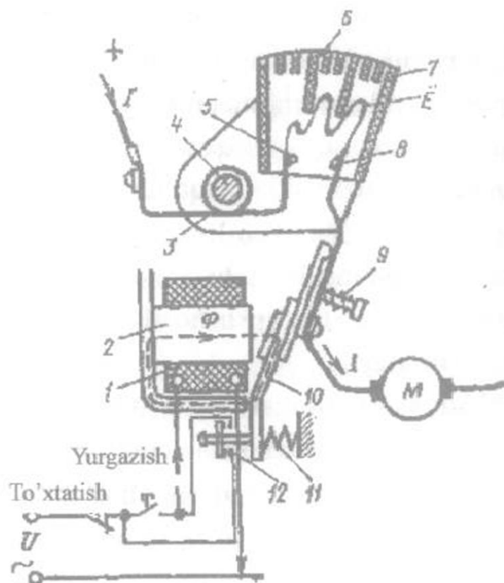
7.5- Rasm. Kontaktorning tuzilishi: 1, 3 - chulg'amlar, 2 - g'altak o'zagi, 4 - magnit bilan puflash o'zagi, 5, 8, 12 - qo'zg'almas, qo'zgaluvchan va yordamchi kontaktlar, 6-izolyatsiyalovchi tusi, 7 - yoy sundiruvchi kamera, 9,11- kontakt prujinasi va qaytaruvchi prujina, 10 - yakor; ye-yoy, M-motor.
