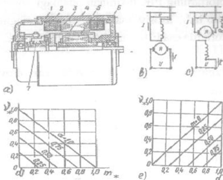
5.40-rasm. Ijrochi o'zgarimas tok motorining umumiy ko'rinishi (a) (bunda: 1 - korpus; 2 - qo'zg'atish chulg'ami; 3 - qutb; 4 - ichi kavak yakor; 5 - ferromagnit o'zak; 6 - podshipnikli qalqon; 7 - kollektor); yakordan (b) va qutbdan (c) boshqariladigani; yakordan boshqariladigan ijrochi motorning mexanik (d) va rostlash (e) xarakteristikalari.
