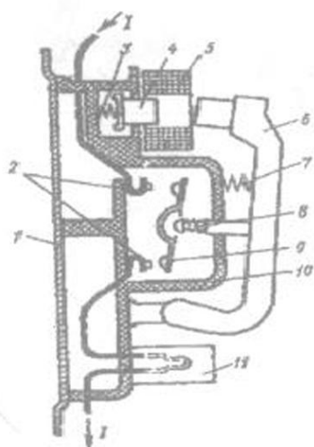
7.7 -Rasm. Burilma yakor yuritgichning tuzilishi: 1-asos, 2,9-qo'zg'almas va qo'zg'aluvchan kontaktlar, 3,7,8-prujinalar, 4-qo'zg'almas magnit o'tkazgich, 5-chulg'am, 6-yakor, 10-izolyatsion kamira, 11-issiqlik relisi
