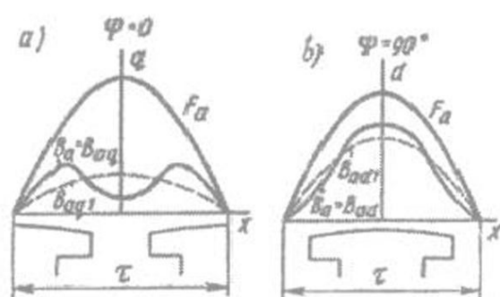
4.6-rasm. Ayon qutbli sinxron mashinaning ko‘ndalang (a) va bo‘ylama (b) o‘qlari bo‘yicha yakor MYKlarining hamda ular osil qilgan magnit induksiylarining taqsimlanish egri chiziqlari
