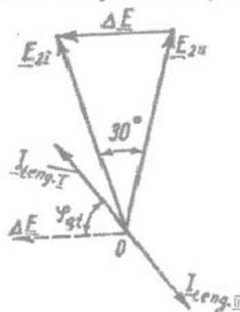
1.22-rasm. Y/Δ - II va Y/Y-0 guruhlariga ega bo'lgan transformatorlarning parallel ishlashida vujudga keladigan tenglashtiruvchi toklar.
