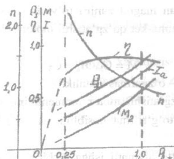
5.28-rasm. Ketma-ket qo'zg'atishli motorning foydali quvvat P_2 ga nisbatan olingan ish xarakteristikalar
