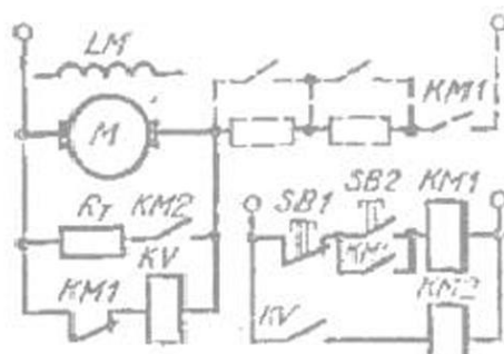
Rasm.7.18 O'zgaras tok motorini EYK funksiyasida avtomatik ishga tushirishning tipik sxemasi.
