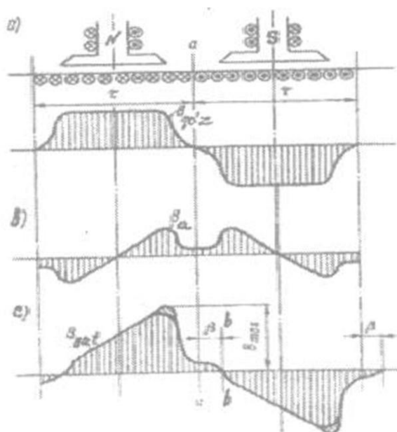
5.13-rasm. Oʻzgarmas tok mashinasining havo oraligʻida magnit induksiyaning taqsimlanishi: a) qoʻzgʻatish chulgʻamining magnit induksiya ( B_{qo'z} ); b) yakor chulgʻamining magnit induksiya ( B_a ); c) mashinaning natijaviy magnit induksiya
