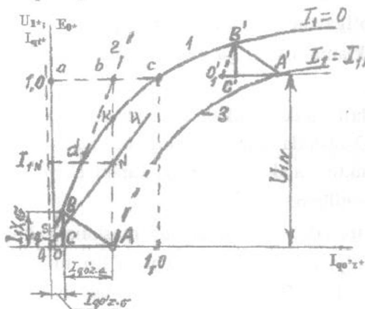
4.11-rasm. Sinxron generatorning: 1 - salt ishlash xarakteristikasi (S.I.X) va 2 - uning boshlan ich (magnit zanjiri to'yinmagan olatdagi, ya'ni to'ri chiziqli) qismini davom qildirib osil qilingan S.I.X; 3 - induksion yuklanish (I.Y.X) va 4 - simmetrik qisqa tutashuv (Q.T.X) xarakteristikalaridan boshlanmay, balki absissalar o'qidagi birorta «A» nuqtadan boshlanadi.
