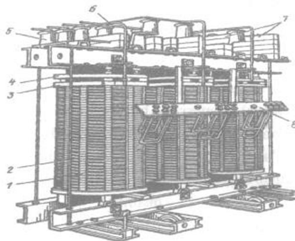
1.6-rasm. Quvvati 320 kV·A bo'lgan quruq kuch transformatorining qoplamasiz ko'rinishi: 1—vertikal tortish shpilkasi; 2—yuqori kuchlanishli chulg'am; 3—chulg'amlarni presslash uchun chinni taglik; 4—presslovchi po'lat halqa; 5—YK ulagichlarning tayanch izolyatorlari; 6—YK ulagichlar; 7—PK ulagichlarni mahkamlash uchun chinni taglik; 8—YK klemma (qisqich)lar taxtasi.
