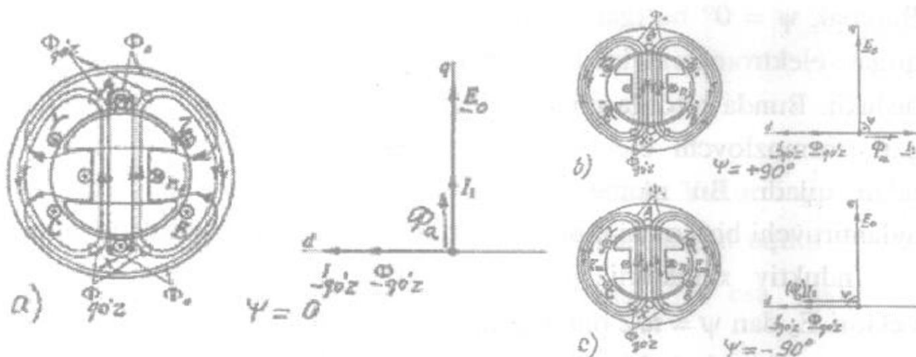
4.7-rasm. Ayon qutbli sinxron generatorning: a - aktiv ( \psi=0 ), b - induktiv ( \psi=+90 ) va c - sig'imiyl ( \psi=-90 ) xarakterli yuklamalardagi yakor reaksiyasi va vektor diagrammalari
