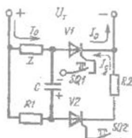
Rasm..7.12 Tiristorli o'zgaras tok kontaktorining sxemasi.
