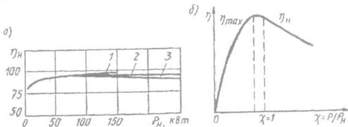
6.11-rasm. Motor quvvatlarini hisoblash va tekshirish uchun: Asinxron matorning f.i.k. ni motor nominal quvvati (a) va yuklamasi karalliligiga bog'liqlik grafiklari (b). 1- A2 seriyali asinxron matorlar; 2- 4A seriyali asinxron motorlar \omega_0 = 157 va 105 rad/s; 3-4A seriyali asinxron matorlar \omega_0 = 314 rad/s.tezligi \omega_N ga bog'liqligi ko'rsatilgan.
