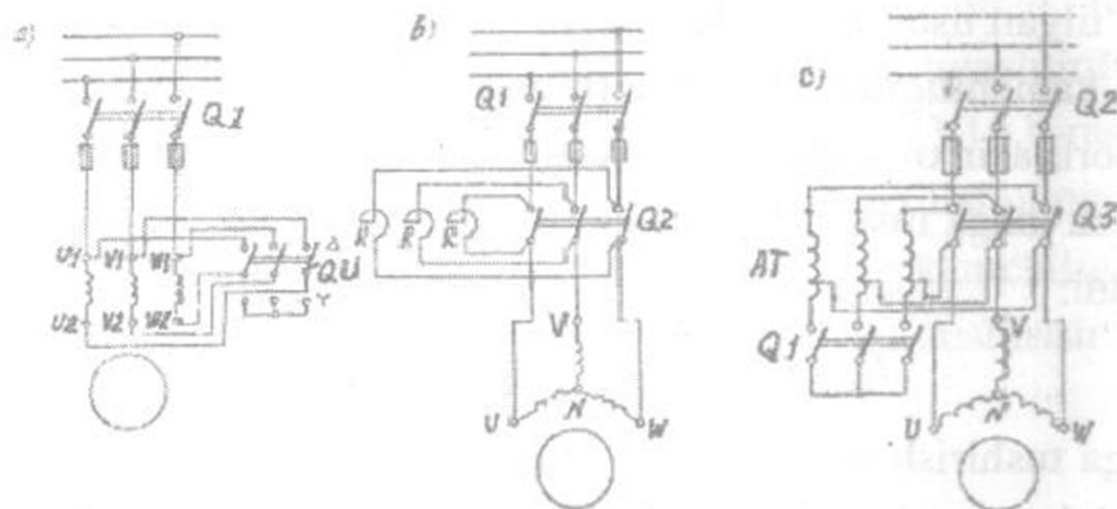
3.15-rasm. Tarmoq kuchlanishini pasaytirib ishga tushirish sxemalari: stator chulg'amini yulduz ulanish sxemadan uchburchak ulanish sxemaga o'tkazish yo'li bilan ishga tushirish (a); stator chul amiga reaktor R (reaktiv qarshilik) ulab (b) yoki AT - avtotransformator yordamida kuchlanishni pasaytirib (s) ishga tushirish sxemalari (bularda: Q_U - qayta ulagich; Q_1 , Q_2 va Q_3 - ishga tushirish kontaktorlari)
