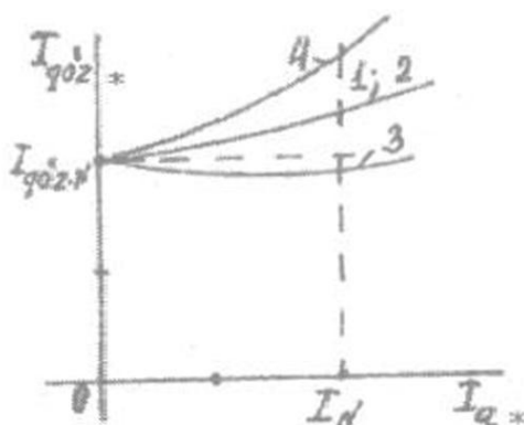
5.23-rasm. Qo'zg'atish cho'lg'amlari har xil sxemalariga xos bo'lgan aralash qo'zg'atishli generatorlarning rostlash xarakteristikalar (1, 2, 3, 4—belgilashlar 24.6- rasmdagilar bilan bir xil).
