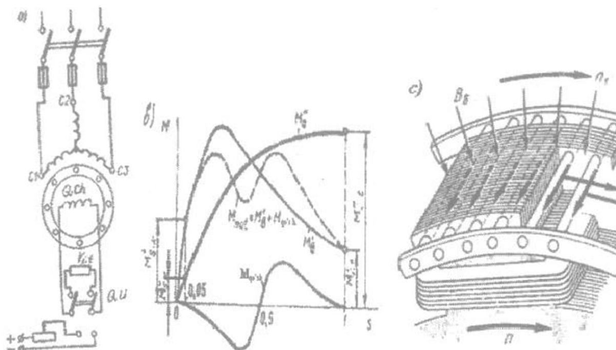
4.22-rasm. Sinxron motorni: a - asinxron usulda ishga tushirish sxemasi va b tushirishdagi asinxron momentlar, bunda: M_a - asosiy moment; M_{qo'sh} - qo'zg'atish ch konturida bir o'qli effekt tufayli vujudga keladigan qo'shimcha moment; M_{s,k} - sinxro kiritish momenti; M_{i,t} - ishga tushirish momenti; F_{em} - ishga tushirish chulg'ami sterjen elektromagnit kuchlar; QCh - qo'zg'atish chulg'ami; QU - qayta ulagich; r_{i,t} - asinxron ishga tushirishda qo'zg'atish chulg'amiga ulanadigan aktiv qarshilik; c - demfer chulg'ar
