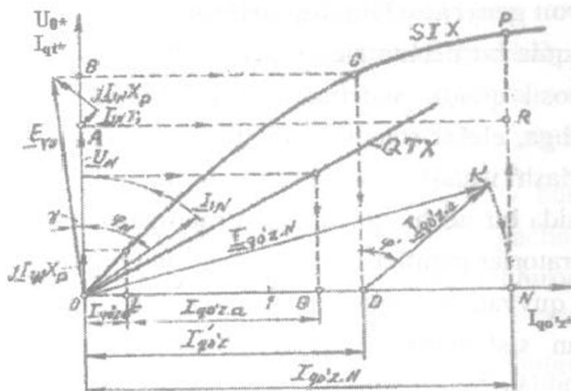
4.13-rasmda SG ning uch xil xarakterli yuklamaga tegishli \cos \varphi qiymatlari uchun rostlash xarakteristiklari ko'rsatilgan.
