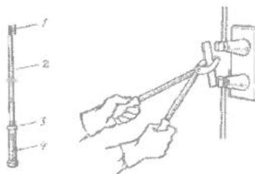
8.3- Rasm. Izolyatsiyalovchi shtanga: 1, 2 - ishlaydigan va izolyatsiyalovchi qismlar, 3 - cheklovchi halqa, 4-dasta
