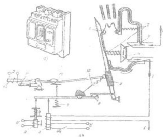
7.8- Rasm. A3700 seriyali avtomatik ajratkich: a-umumiy ko'rinishi, b - prinsipial sxemasi; 1- uzuvchi kontakt, 2, 7, 13 - prujinalar, 3, 4 - asosiy (bosh) kontaktlar, 5 - ko'taruvchi detal, 6 - ilgak, 8, 9 - maksimal va minimal ajratkichlar g'altaklari, 10 -elektromag-nit, 11- dasta, 12 -richaglar
