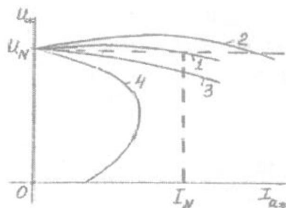
5.22-rasm. Aralash qo'zg'atishli generatorning tashqi xarakteristikalari (1; 2; 4); 3 – parallel qo'zg'atishli uchun (taqqoslash uchun keltirilgan).
