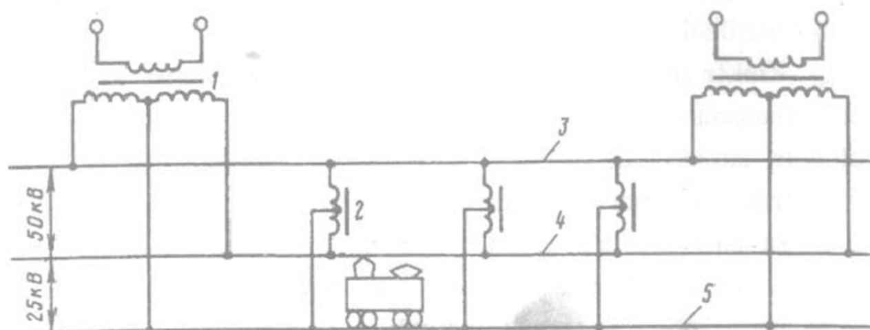
1.29-rasm. Elektrlashtirilgan temir yo'lining 2x25 elektr ta'minoti tizimi tortish nimstansiyasidagi ikkilamchi chulg'am bo'lingan bir fazali maxsus maqsadli kuch transformatori: (1 - bir fazali kuch transformatori; 2 - bir fazali kuch AT; 3 - elektr energiyani ta'minlovchi maxsus liniya; 4 - kontakt tarmog'i; 5 - rels tarmog'i).
