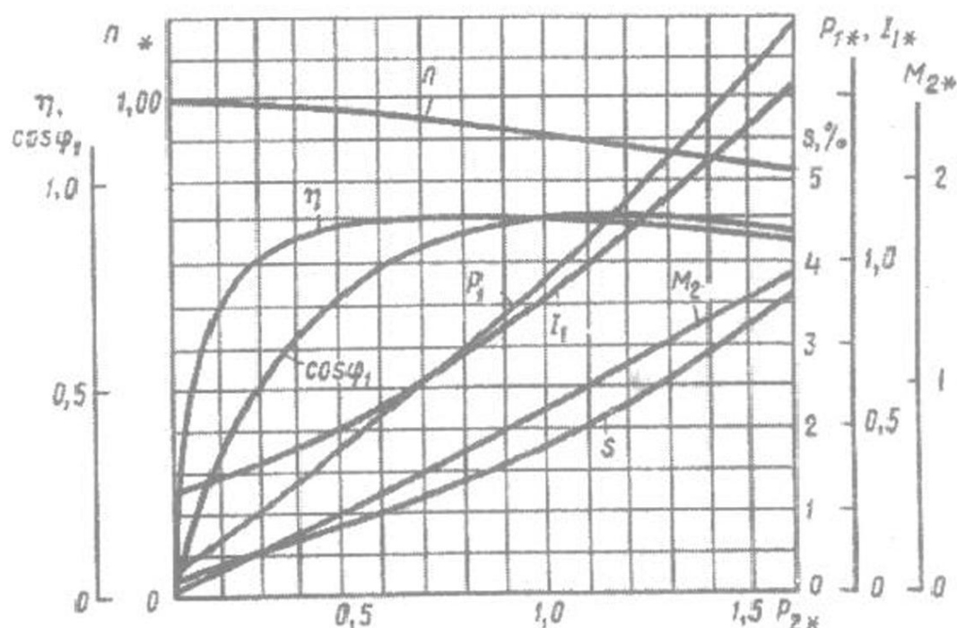
3.13-rasm. Quvvati 50 kW, 220/380 V, 1470 ayl./min bo'lgan qicqa tutashgan rotorli asinxron motorning ish xarakteristikallari
