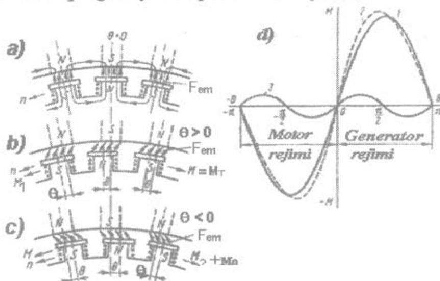
4.19-rasm. Qo'zg'atish chulg'ami magnit oqimi \Phi_{qo'z} va stator chulg'ami natijaviy magnit oqimi \Phi_{nat} larning sinxron mashina salt ishlashida (a), generator (b) va motor (c) rejimlarida o'zaro ta'siri natijasida burchakning hosil bo'lishi hamda motor va generator rejimlari uchun burchak xarakteristikalar
