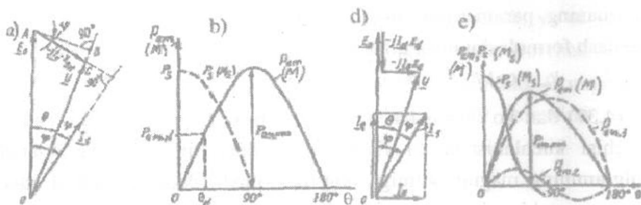
4.15-rasm. Ayon bo'lmagan qutbli (a, b) va ayon qutbli (d, e) SGning elektromagnit quvvatini aniqlashga oid soddalashtirilgan vektor diagrammalar (a, d) va tegishli aktiv quvvatining burchak xarakteristikalar (b, e).
