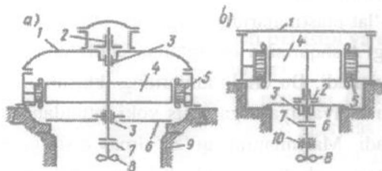
4.3-rasm. Gidrogeneratorlarning konstruktiv sxemalari - osma (a) va soyavon (b) tiplari:
