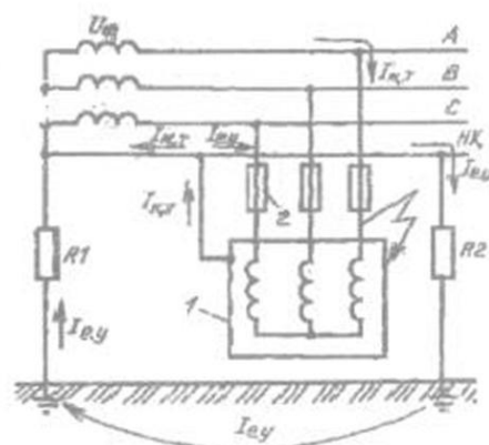
8.2- Rasm. Himoyalash uchun nol simga ulash sxemasi: 1 - elektr qurilma, 2 - saqlagichlar, R1 va R2 - yerga ulovchi rezistorlar, I_{eu} - yerga ulash toki. U_\phi - faza kuchlanishi
