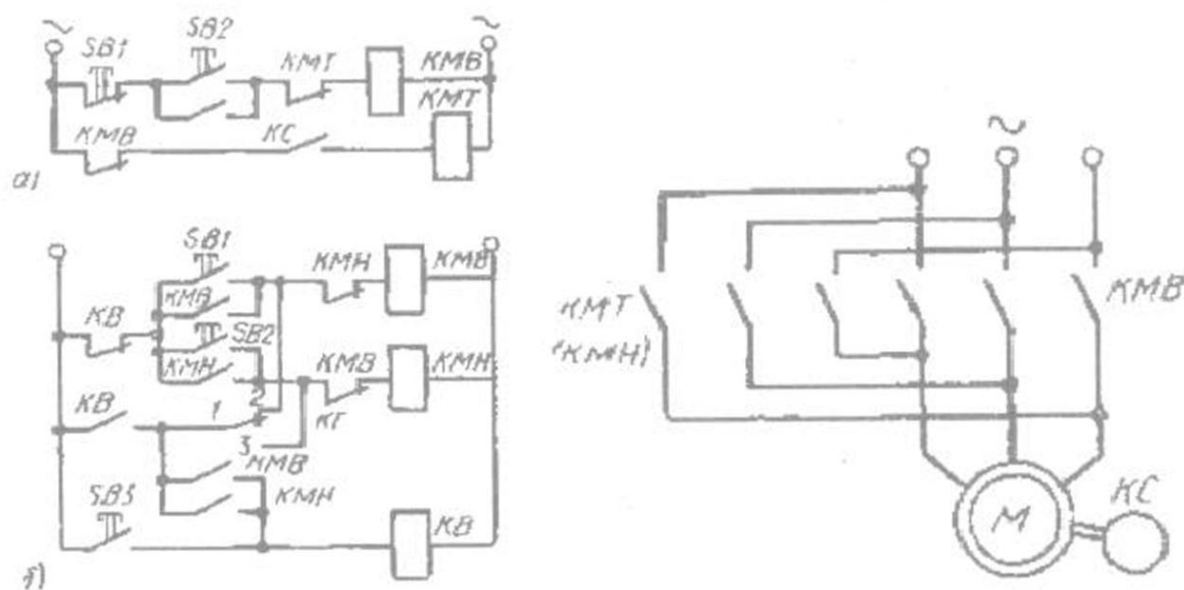
Rasm.7.20 Tezlikni nazorat qiluvchi relesi bo'lgan asinxron matorni tormozlash sxemalari: a - motorni noreversiv boshqarish sxemasi, b - motorni reversiv boshqarish sxemasi.
