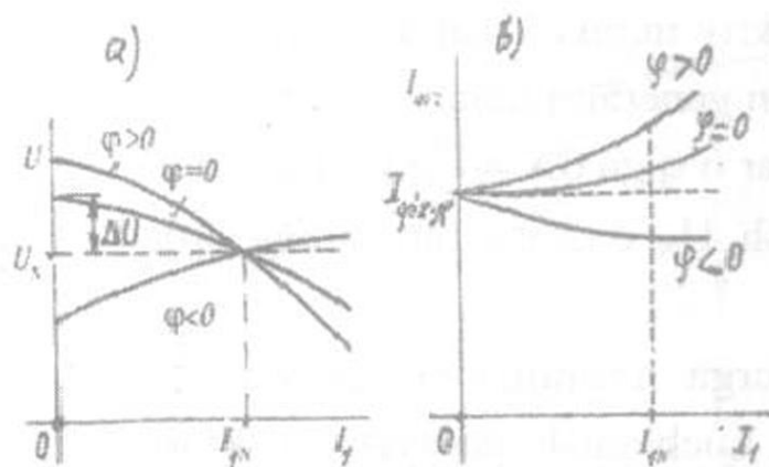
4.12-rasm. Sinxron generatorning yuklamasini kamaytirib olingan tashqi (a) va yuklamasini oshirib olingan rostlash (b) xarakteristikalar (bular: \varphi_0 - aktiv, > 0 - aktiv-induktiv va < 0 - aktiv-sig'imiyl xarakterli yuklamalarga xos).
