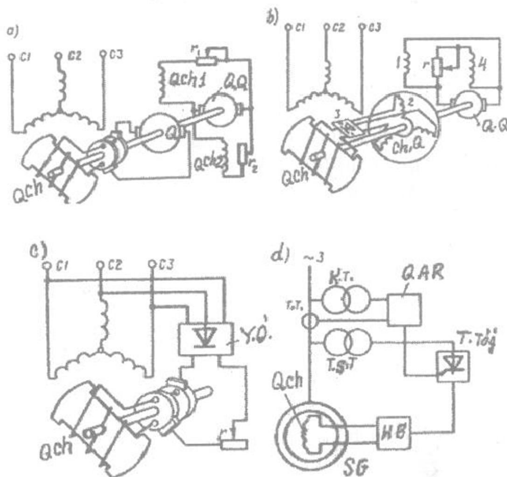
4.4-rasm. Sinxron generatorlarni elektromagnit qo'zg'atishning: a - kontaktli tizimi (bunda: QCh - SG ning qo'zg'atish chulami, Q - qo'zg'atgich, Q.Q - qo'zg'atgichning qo'zg'atgichi, QCh1 va r_1 - qo'zg'atgichning qo'zg'atish chulami va rostdash reostati, QCh2 va r_2 - Q.Q ning qo'zg'atish chulg'ami va rostdash reostati) va b - kontaksiz (bunda: Ch.Q - cho'tkasiz qo'zg'atgich va uning: 1 - qo'zg'atish va 2 - yakor chulg'amlari, 3 - yarim o'tkazgichli to'g'rilagich); c - o'z-o'zini qo'zg'atish prinsipiga oid chizma (bunda: YO' - yarimo'tkazgich; r - rostdash reostati); d - o'z-o'zini qo'zg'atish avtomatik tizimsining strukturali sxemasi (bunda: KT - kuchlanish transformatori, T.T - tok transformatori, T.S.T - to'g'rilagich sxemaning transformatori, QAR - qo'zg'atishni avtomatik rostdash qurilmasi, T.To'g' - tiristorli to'g'rilagich, HB - himoya bloki, SG - sinxron generator)
