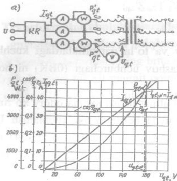
1.15- rasm. Quvvati S_{Nq} = 100 kVA; U_{1N} / U_{2Nq} 6,3 / 0,22 kV; chulg'amlari Y/Y ulangan, uch fazali ikki chulg'amli transformatorning qisqa tutashuv tajribasini o'tkazish sxemasi (a) va qisqa tutashuv xarakteristiklari (b); K.R - kuchlanishni rostlagich
