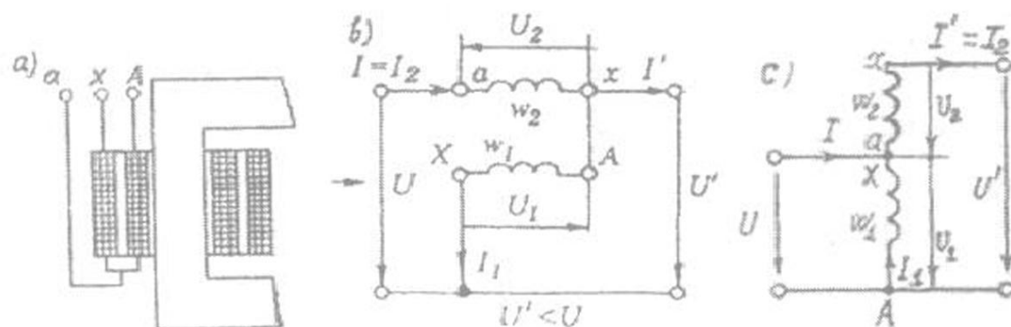
1.26.-rasm. Katta quvvatli AT o'zgida chulg'amlarning joylashtirilishi (a) va oshiruvchi AT ning prinsipial sxemasi (b) hamda chulg'amining bir qismi ikkilamchi chulg'am vazifasini bajaradigan kam quvvatli bir fazali pasaytiruvchi AT ning prinsipial sxemasi (c).
