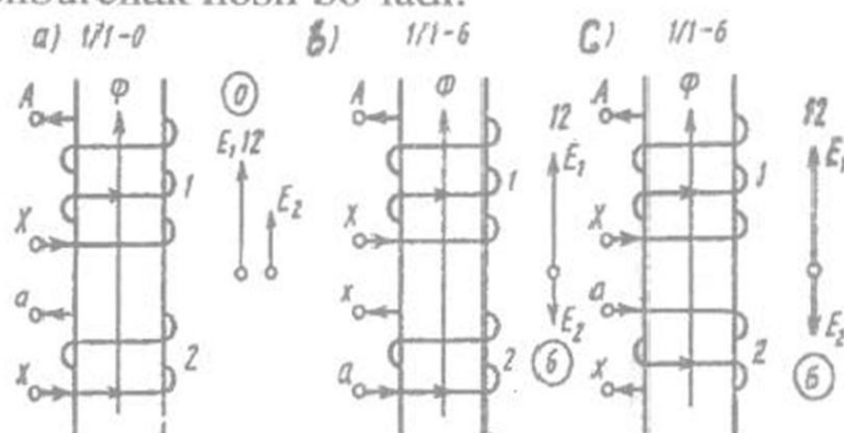
1.16-rasm. Bir fazali transformator chulg'ami ulash guruhleri
