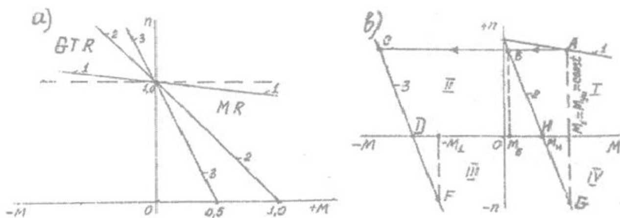
5.38-rasm. Parallel qo'zg'atishli motorning: rekuperativli (generatorli) (a) va teskari ulash yo'li bilan (b) tormozlashdagi mexanik xarakteristikalar; GTR - generatorli tormozlash rejimi; MR - motor rejimi.
