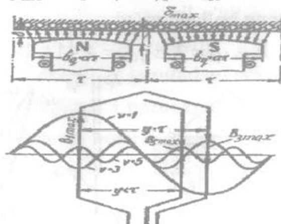
2.12-rasm. Ayon qutbli sinxron generatorda o'zgatish chulg'ami hosil qilgan magnet maydon induksiyasi garmonikalarining mashina havo oralig'idagi stator yuzasi bo'ylab taqsimlanishi; bq – qutb uchligi kengligi.
