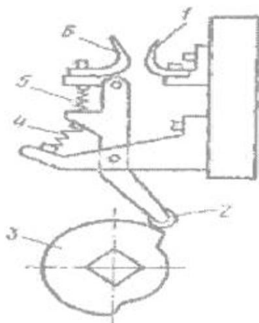
Rasm.7.4 Kulachokli kontrollerning seksiyasi 1, 6 -qo'zg'almas va qo'zgaluvchan kontaktlar, 2-rolik, 3-kulachok, 4,5-prujinalar
