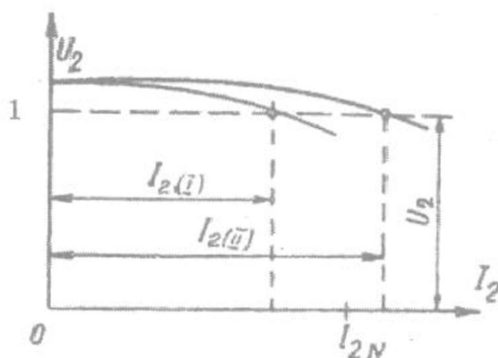
1.21-rasm. Qisqa tutashuv kuchlanishlari bir xil bo'lmagan holda parallel ishlayotgan ikkita transformatorning tashqi xarakteristikalarini yordamida yuklama taqsimlanishini aniqlash.
