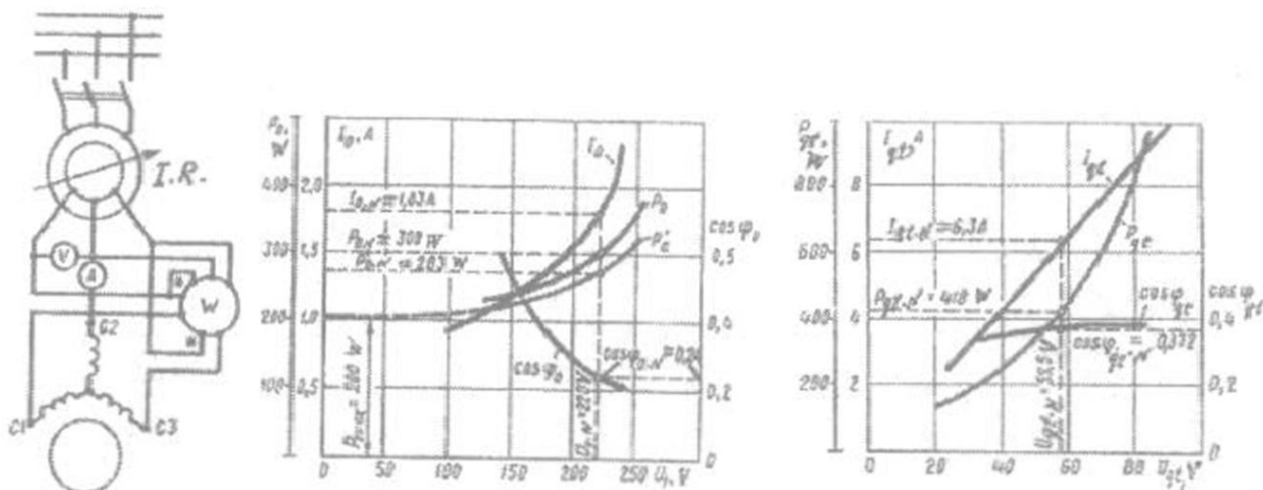
3.11-rasm. Uch fazali asinxron motor (3 kW, 220/380 V, 1430 ayl/min) ning salt ishlash va qisqa tutashuv tajribalarini o'tkazish sxemasi (a); salt ishlash (b) va qisqa tutashuv (s) xarakteristikalarini; I.R. - induksion regulyator; \Delta P_{0,N} -nominal kuchlanishdagi magnit va mexanik isroflar yig'indisi
