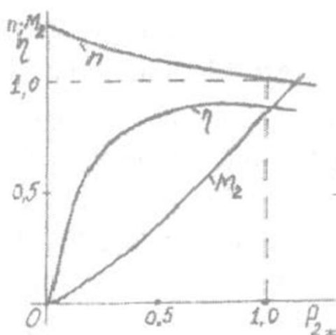
5.29-rasm. Mos ulangan aralash qo'zg'atishli motorning ish xarakteristikalar (asosiy chulg'am - parallel qo'zg'atishli, qo'shimcha chulg'am ketma-ket qo'zg'atishli).
