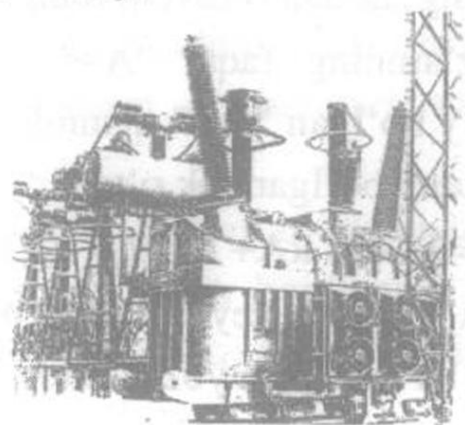
1.24-rasm. Elektr energetikasi tizimida ekspluatatsiya uchun o'rnatilgan katta quvvatli yuqori kuchlanishli bir fazali avtotransformator.
