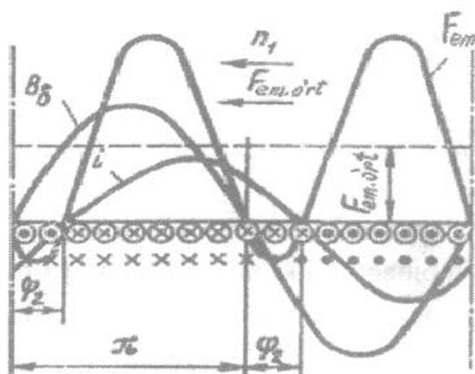
3.6-rasm. Mashina havo oralig'ining magnit induksiyasi ( B_\delta ), rotor chulg'ami toki ( i ) va asinxron mashina chulamlari o'tkazgichlariga ta'sir qiladigan elektromagnit kuch ( F_{em} ) larning taqsimlanish egri chiziqlari
