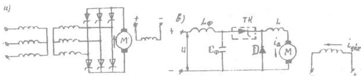
5.35-rasm. Boshqariladigan to'g'rilagichdan ta'minlanadigan mustaqil qo'zg'atishli motorning aylanish chastotasini rostlash sxemasi (a) va o'zgaras tok motorini impulsli rostlash (b):
