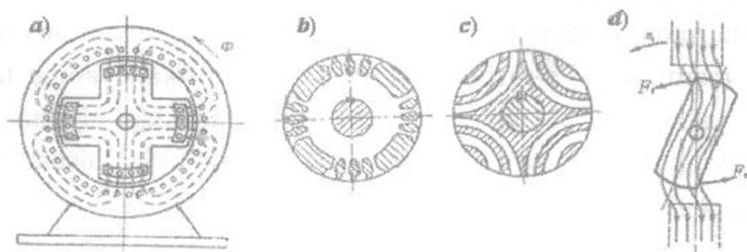
4.27-rasm. To'rt qutbli ishga tushirish (dempfer) chulg'amli ayon qutbli sinxron reaktiv motorning odatdagi magnit o'tkazgich konstruksiyasi (a) va uning noayon ko'rinishdagi modifikatsiyasi (b); takomillashtirilgan, ya'ni mashinaning ko'ndalang o'qi bo'yicha induktiv qarshiligi x_q ni kamaytirish maqsadida nomagnit oraliqlarga quyma aluminiy sterjenlardan hosil qilingan dempfer chulg'amli segmentlangan magnit o'tkazgich (c) va ikki qutbli sinxronmotor uchun reaktiv momentning vujudga kelish sxemasi (d); F_t – tangensial kuch.
